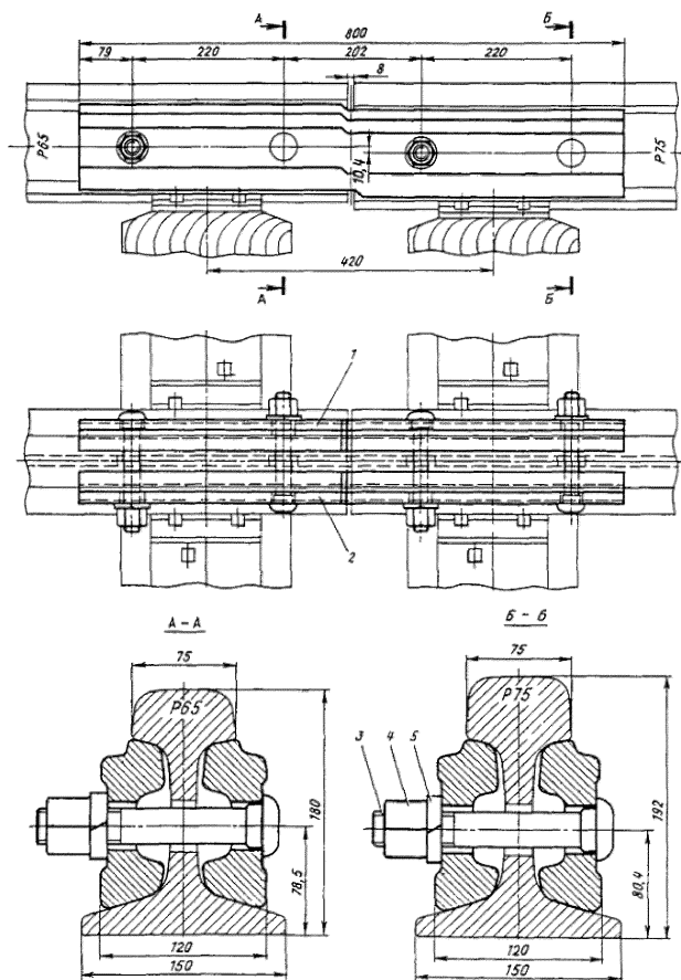
Рисунок 6.2 – Переходный стык рельсов Р75–Р65
