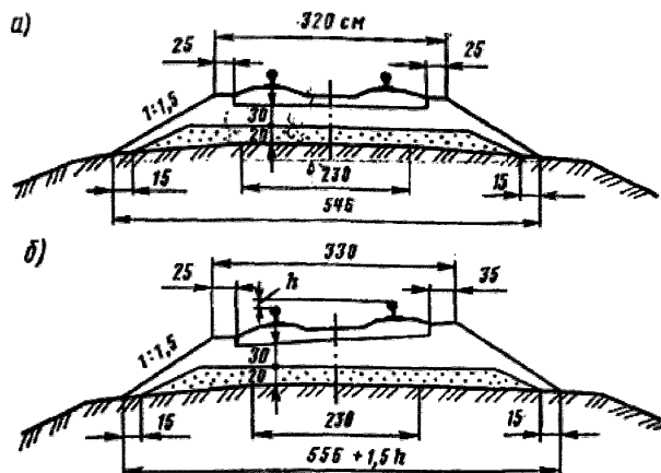
Рисунок 6.25 – Поперечные профили балластного слоя для пути легкого типа с железобетонными шпалами однопутных линий: а – прямой участок; б – кривая
