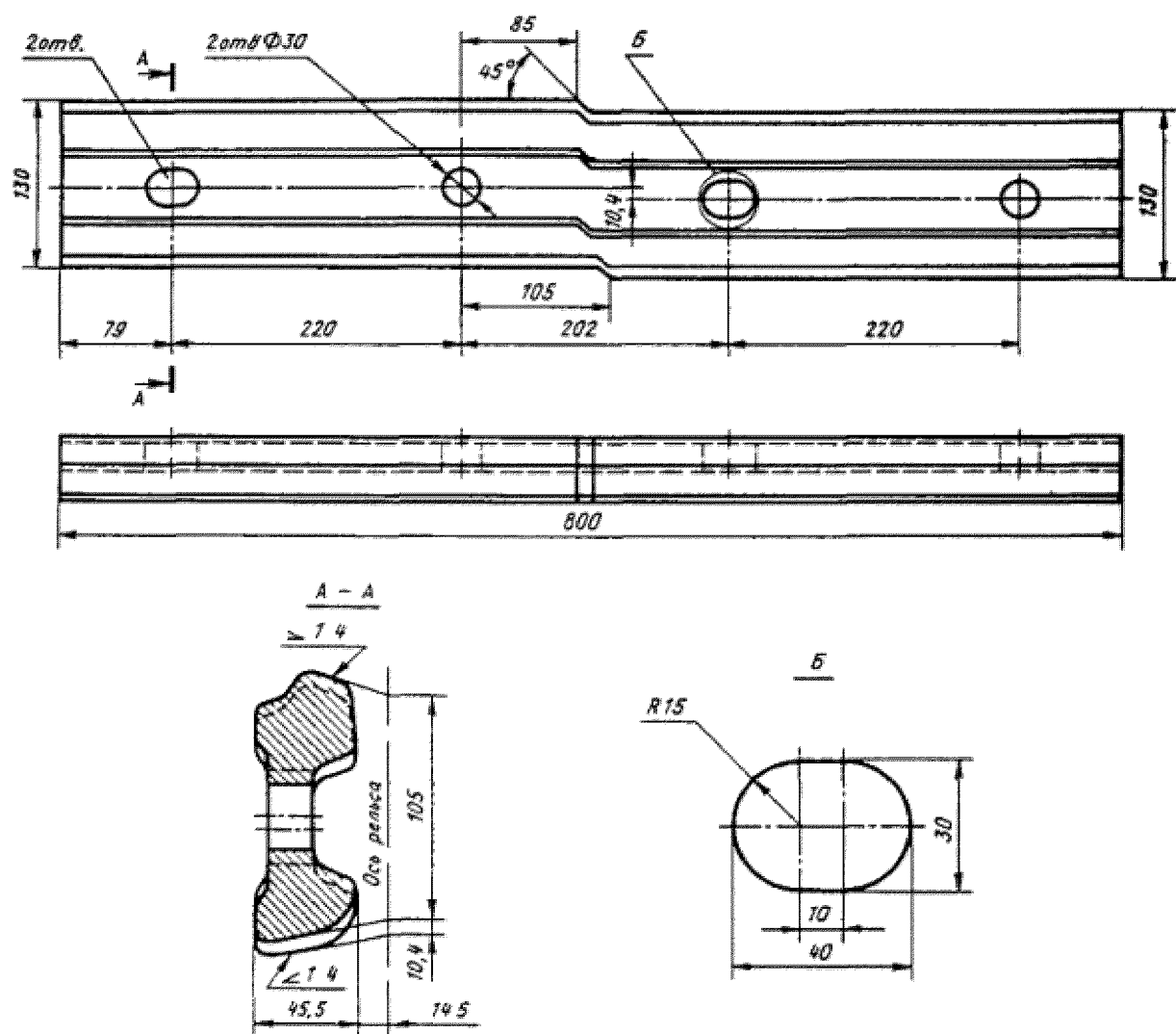
Рисунок 6.1 – Накладка переходная Р75–Р65 (левая)
