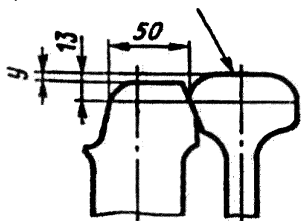
Рисунок 6.49 – Измерение понижения остряка относительно рамного рельса y :
