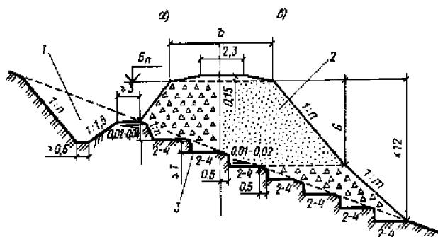
Рисунок 6.32 – Конструкции насыпей:
