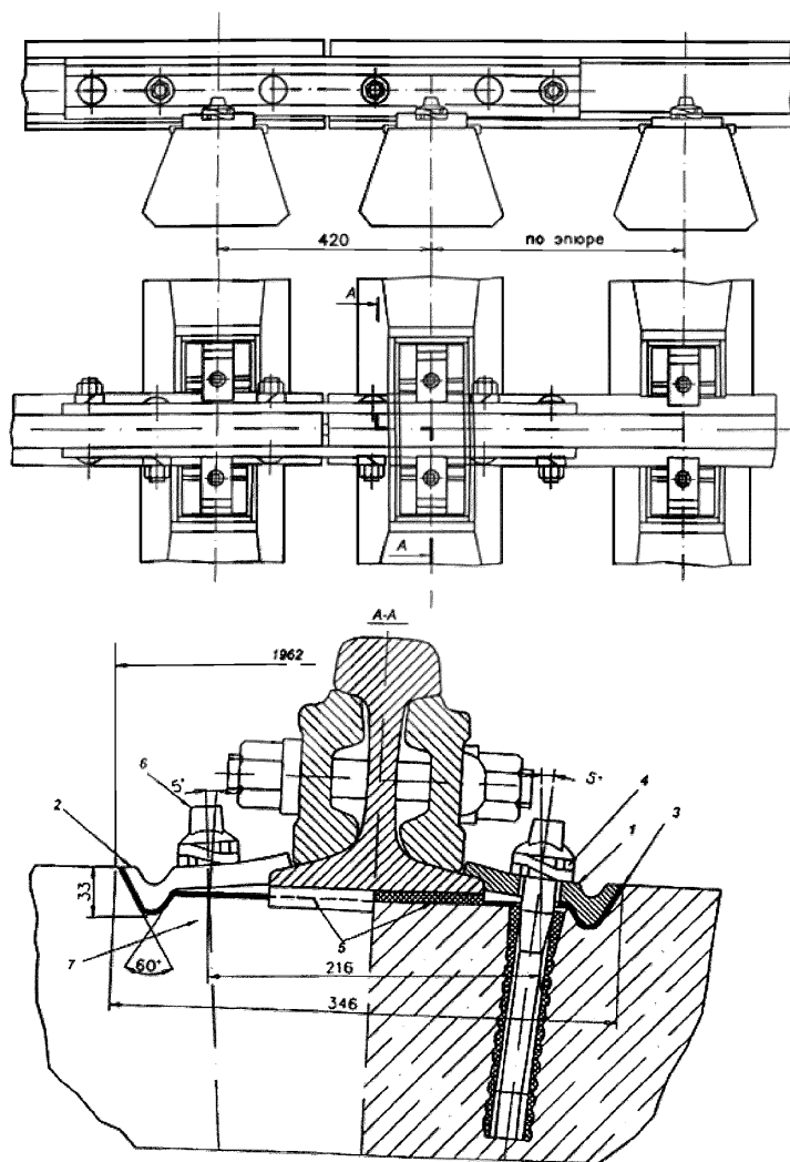
Рисунок 6.14 – Стыковое и промежуточное шурупно-дюбельное крепление типа ШД-65 на железобетонных шпалах типа ШСП-Д с рельсами Р65:
