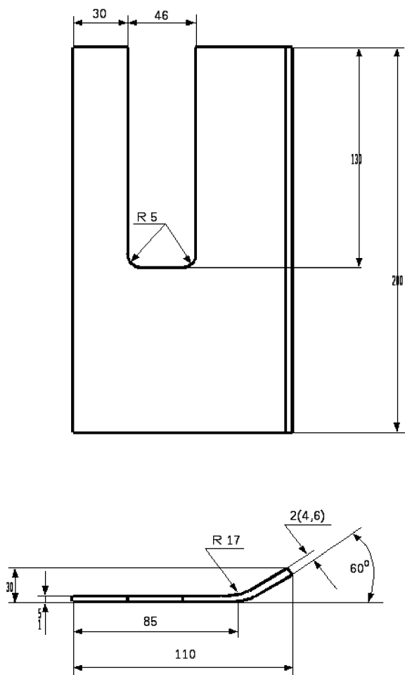
Рисунок 6.39 – Специальная прокладка из изолирующего материала для регулировки ширины колеи
