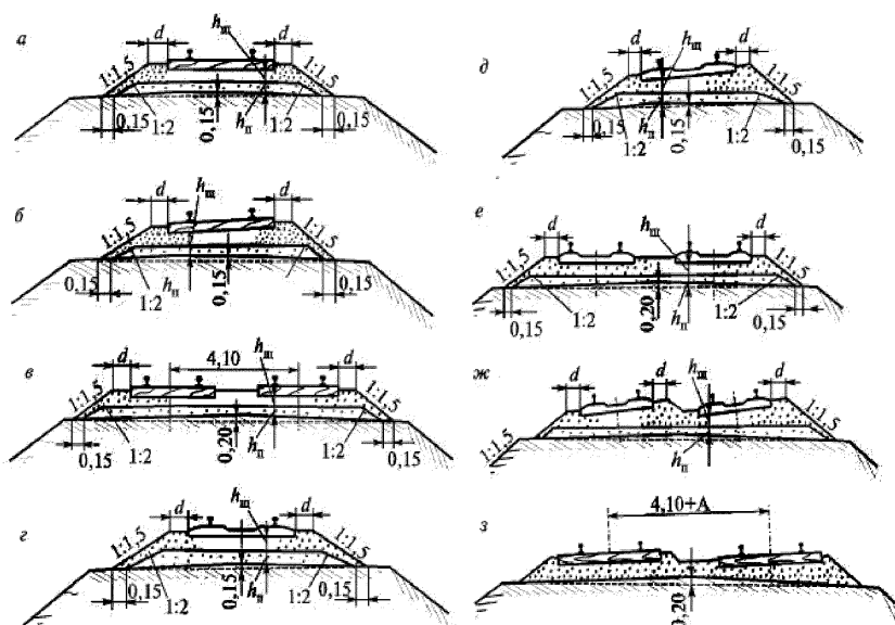
Рисунок 6.24. Поперечные профили балластной призмы:
