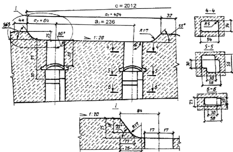
Рисунок 6.18 – Подрельсовая часть шпалы ШП-2-1
