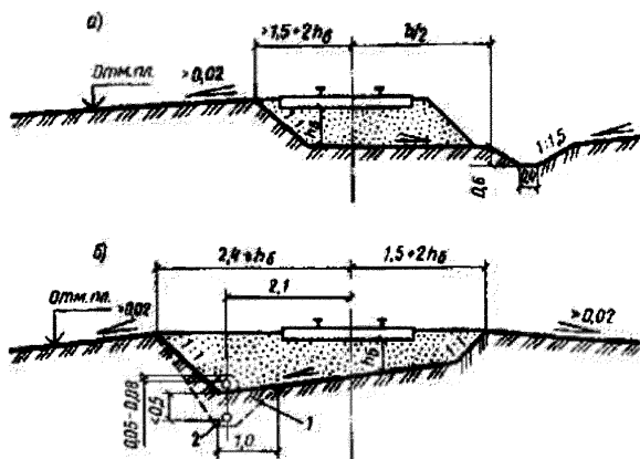
Рисунок 7.29 – Конструкции земляного полотна:
