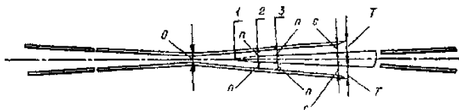
Рисунок 6.47 – Места контрольных измерений ширины желобов в острой крестовине:
