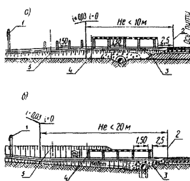
Рисунок 8.1 – Продольный профиль переезда (размеры даны в метрах): а – на насыпи; б – в выемке; 1 – знак «Берегись поезда»; 2 – место крайнего рельса; 3 – дренажная призма; 4 – ось шлагбаума; 5 – ось габаритных ворот на электрифицированных линиях
