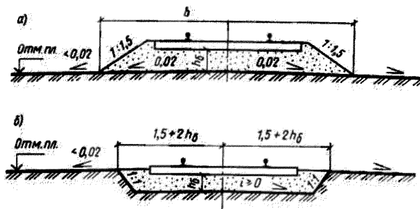
Рисунок 7.30 – Конструкции земляного полотна:
