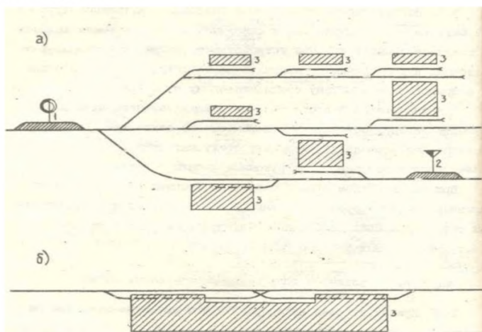
Рисунок 5.1 – Схема примыкания погрузочно-разгрузочных путей к соединительным путям:
