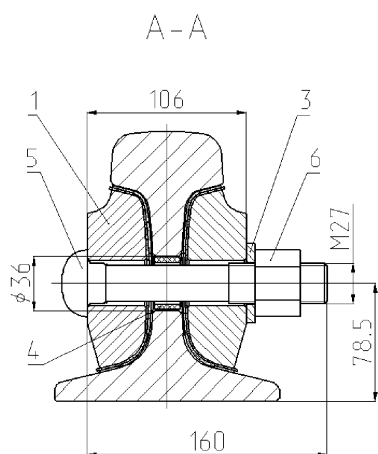
Рисунок 6.13 – Стык, изолирующий рельсов типа Р65 с комбинированными (металлокомпозитными) накладками
