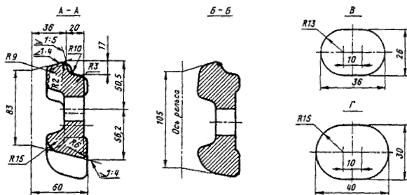
Рисунок 6.6 – Накладка переходная P65–P50 (правая)
