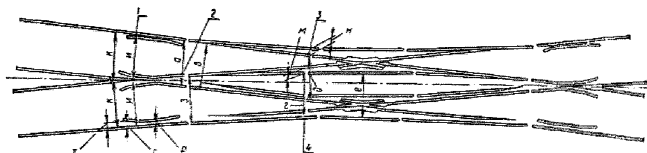
Рисунок 6.45 – Места контрольных измерений ширины колеи на двойных перекрестных стрелочных переводах и желобов на стрелке и в контррельсах
