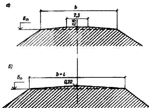
Рисунок 7.28 – Конструкция верха железнодорожного земляного полотна:
