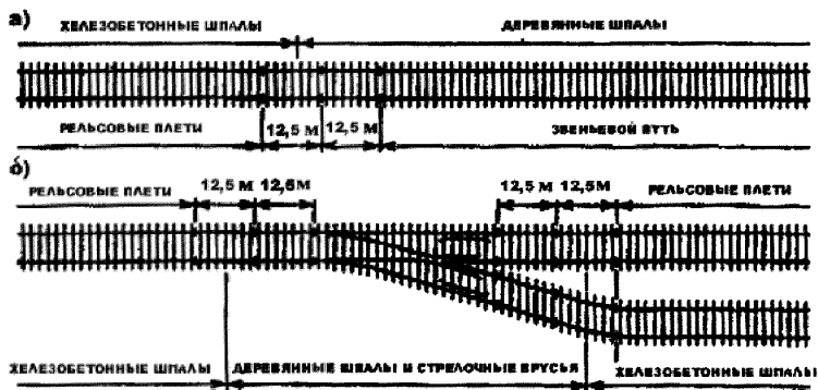
Рисунок 6.33 – Схемы примыкания бесстыкового пути на железобетонных шпалах:
