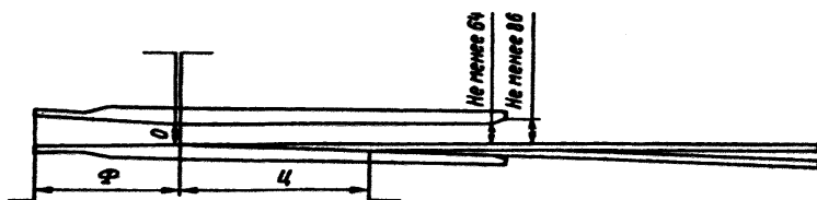
Рисунок 6.41 – Места контрольных измерений ширины желобов и расстояний от переднего торца усовика до переднего торца длинного рельса сердечника (Φ) и между торцами длинного и короткого рельса сердечника (Ц) на крестовина с подвижным сердечником
