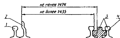
Рисунок 6.46 – Схема измерения расстояний между рабочими гранями контрольного рельса и усовика и рабочими гранями контрольного рельса и сердечника крестовины (размеры даны в мм)
