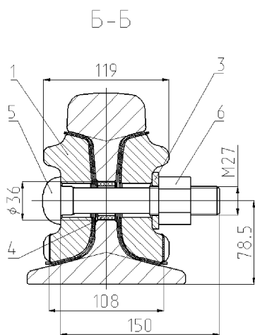
Рисунок 6.13 – Стык, изолирующий рельсов типа Р65 с комбинированными (металлокомпозитными) накладками
