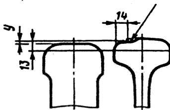
Рисунок 6.49 – Измерение понижения остряка относительно рамного рельса y :
