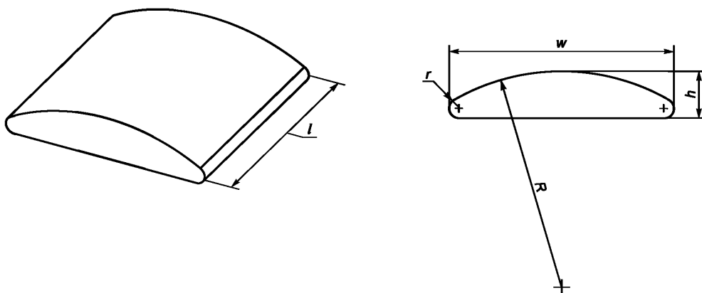
Рисунок 9 — Нагрузочная подушка для тазовой части (размеры приведены в таблице 1)
