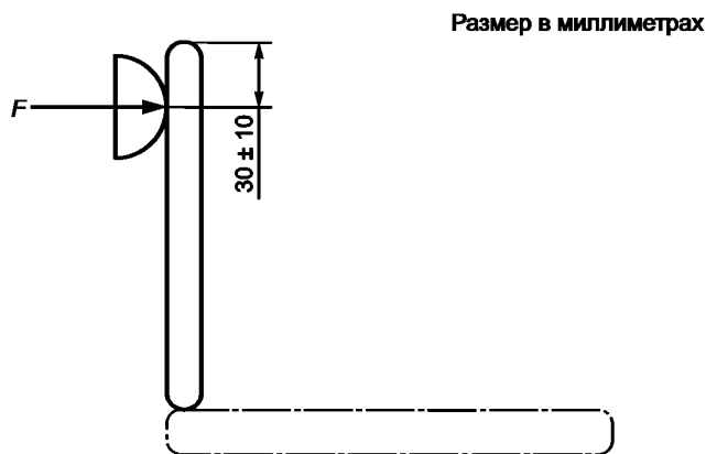
Рисунок 21 — Пример приложения силы спереди к опоре спины
