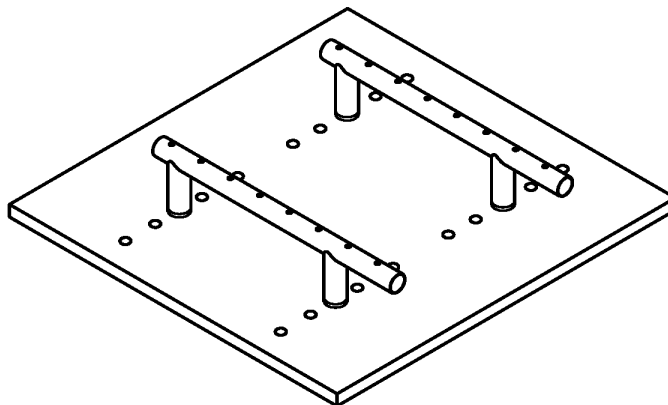
Рисунок 4 — Пример регулируемой жесткой испытательной рамы
