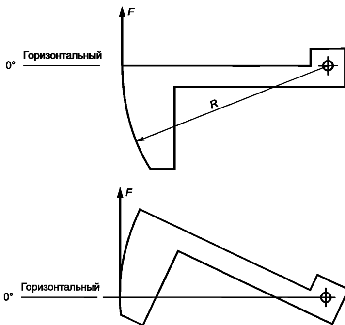
Рисунок 6 — Пример поворотной испытательной рамы
