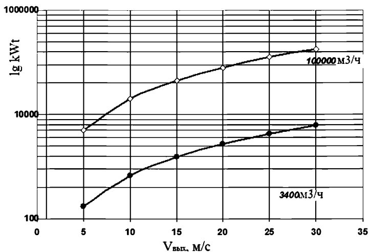
Рисунок 6.2 – Энергетические затраты при выходе воздуха в атмосферу
