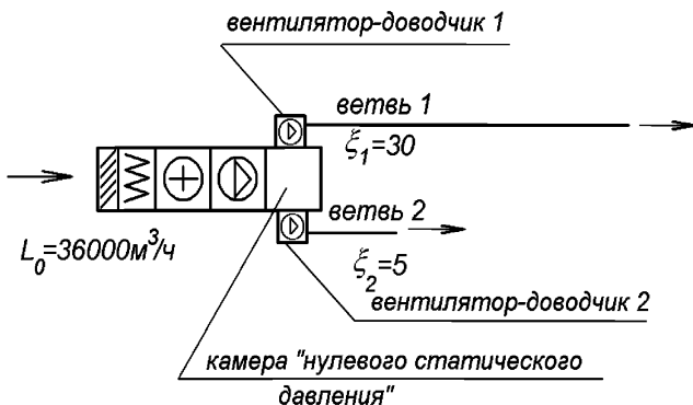
Рисунок Ж.6 – Вентсистема с «камерой нулевого статического давления» и «вентиляторами–доводчиками» в каждой ветви.
