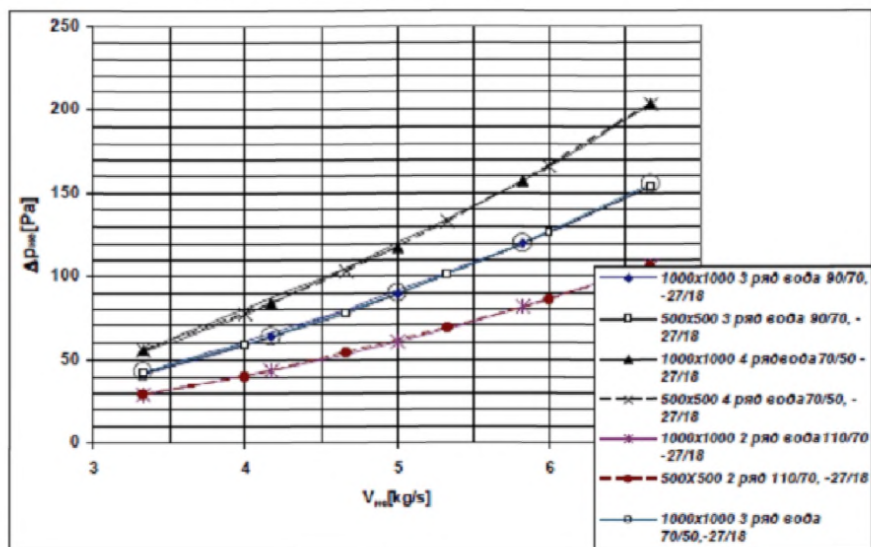
Рисунок 6.1 – «Нормативные» потери в медно-алюминиевых воздушно-водяных теплообменниках для нагрева воздуха
