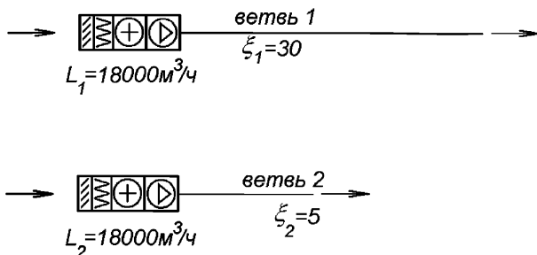
Рисунок Ж.4 – Две независимых вентсистемы
