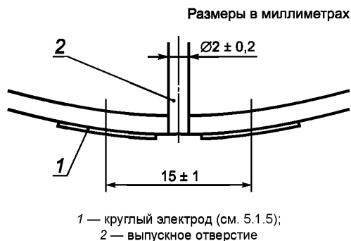
Рисунок 2 — Поперечный разрез А—В
