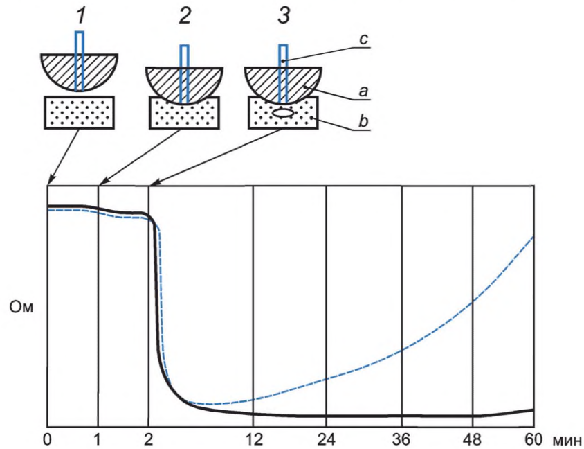
1 — начало измерения импеданса; 2 — начало нагрузки 500 N; 3 — начало вливания жидкости; а — нагрузочный индентор для определения защиты от пота для жесткой подушки; b — подушка; с — сливной механизм
