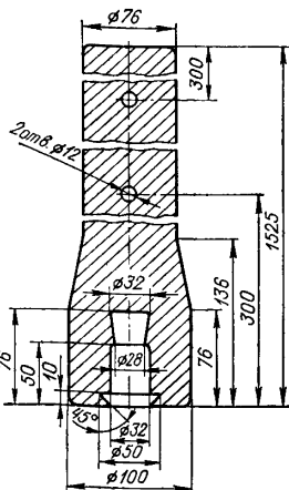
Рис. 10. Электрод железокремнистый, тип З.
