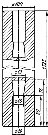
Рис. 11. Электрод железокремнистый, тип И.
