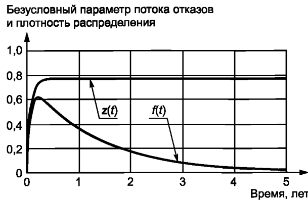
Рисунок 30 — Графики зависимости от времени z(t) и f(t)
