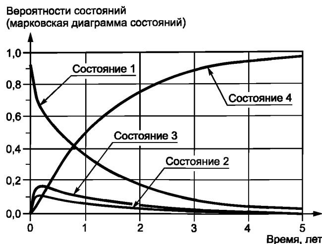
Рисунок 25 — График зависимости от времени вероятностей состояний для марковской модели, представленной на рисунке 24
