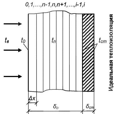
Рис. 2. Схема к расчету на ЭВМ прогрева стальной пластины с огнезащитной облицовкой.
