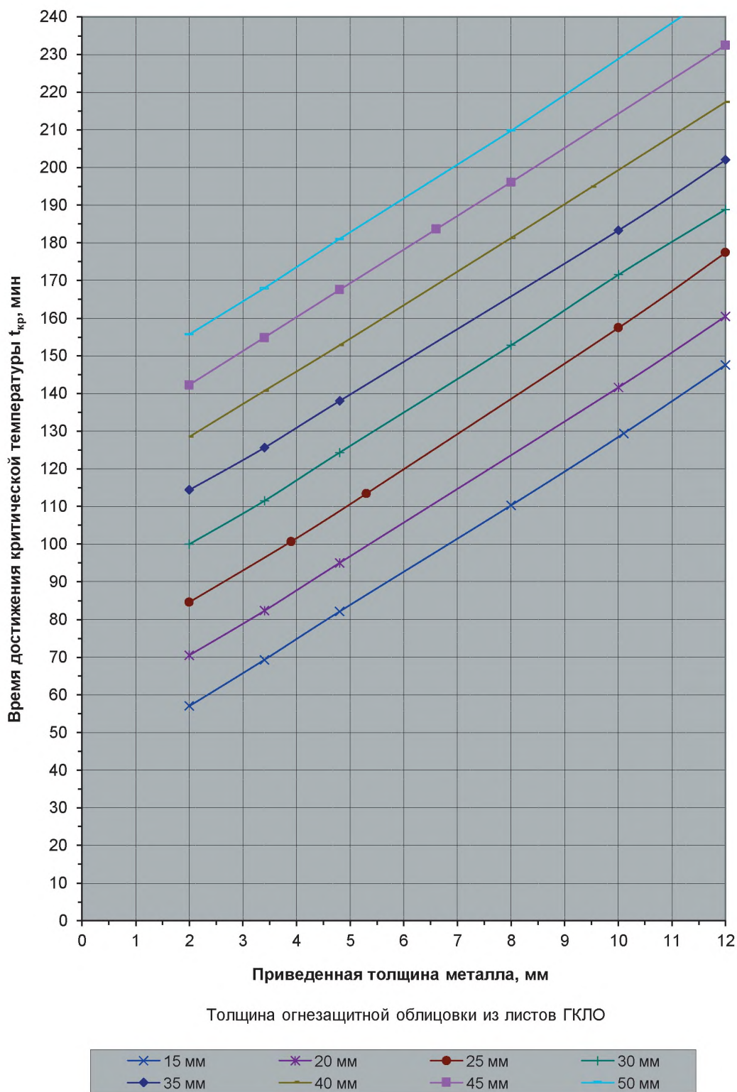
Рис. 14. Огнестойкость стальных конструкций с огнезащитной облицовкой Из листов ГКЛО при t_{кр} = 600^\circ\text{C}
