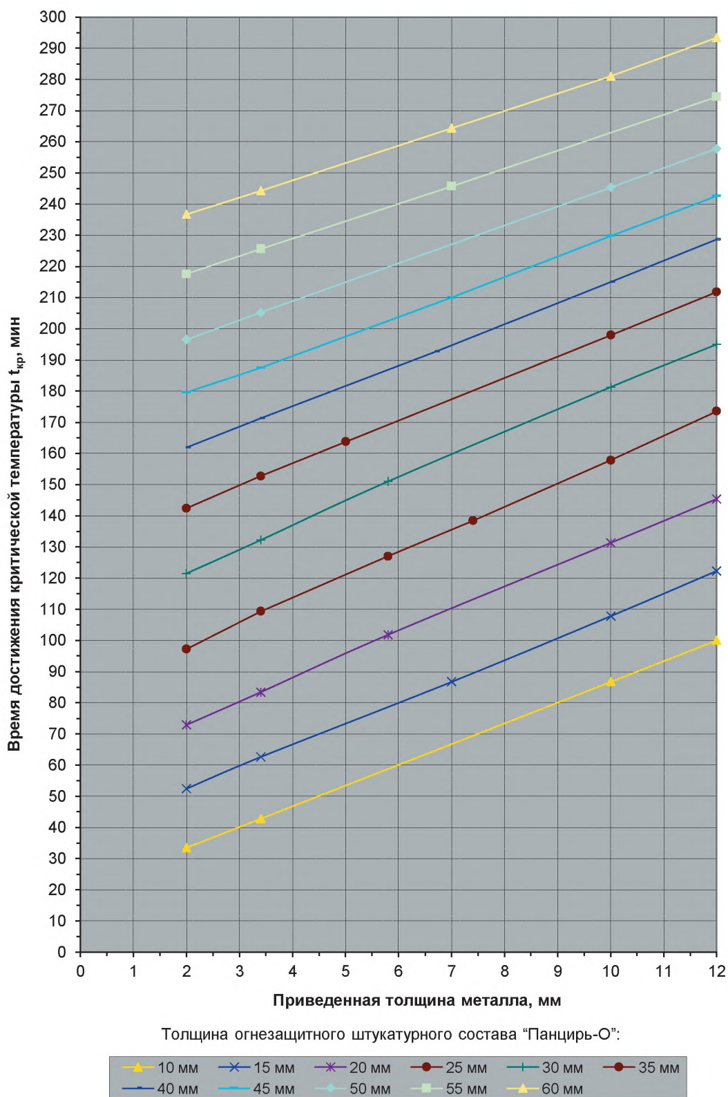
Рис. 20. Огнестойкость стальных конструкций с огнезащитным штукатурным составом «Панцирь-О» при t_{кр} = 500^\circ\text{C} .
