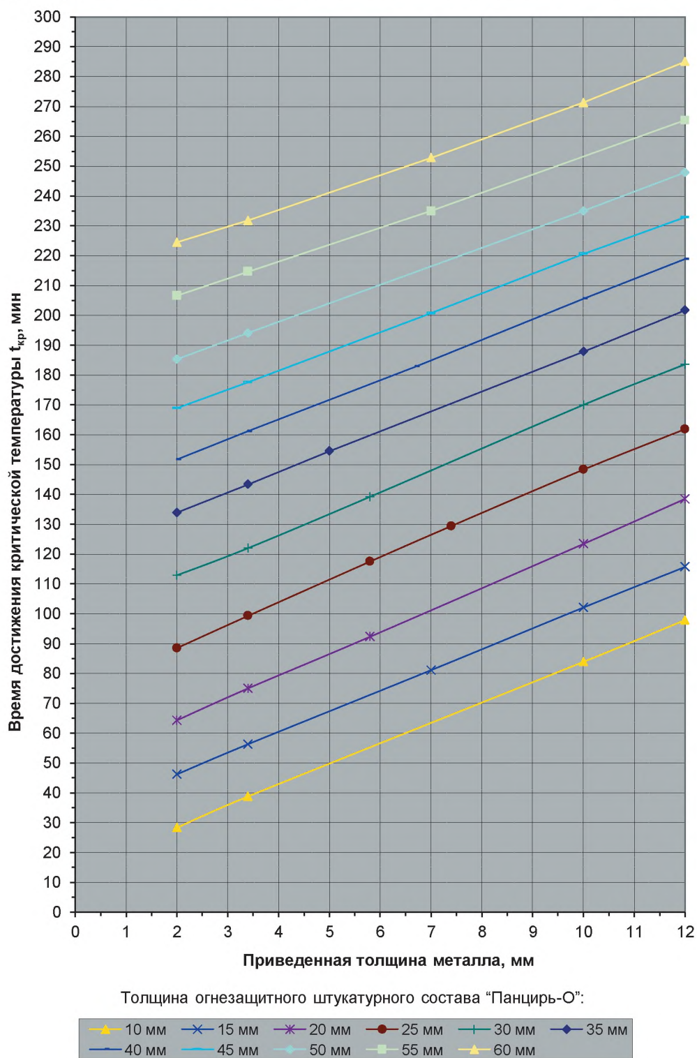
Рис. 19. Огнестойкость стальных конструкций с огнезащитным штукатурным составом "Панцирь-О" при t_{кр} = 450^\circ\text{C} .
