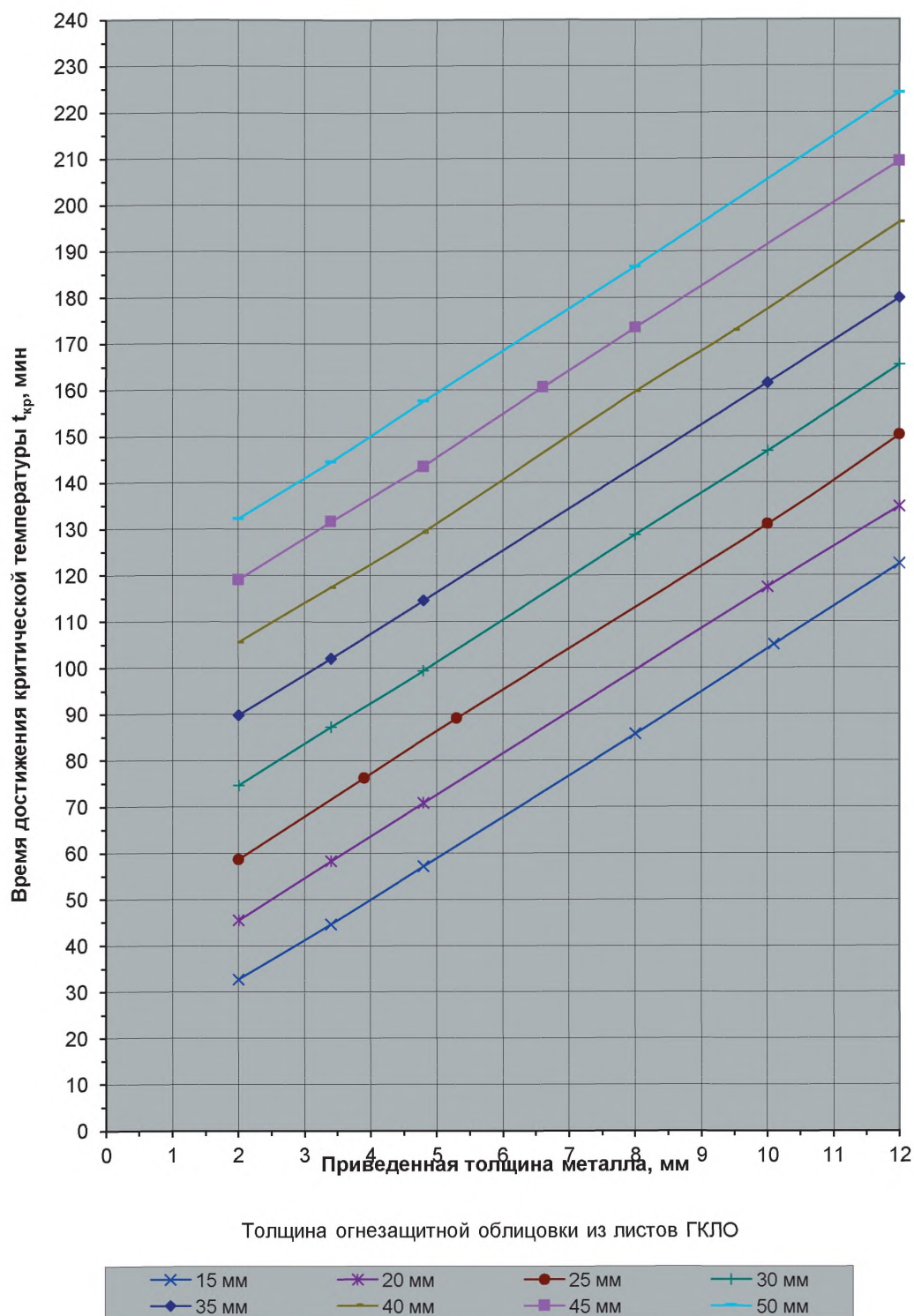
Рис. 11. Огнестойкость стальных конструкций с огнезащитной облицовкой из листов ГКЛО при t_{кр} = 450^\circ\text{C}
