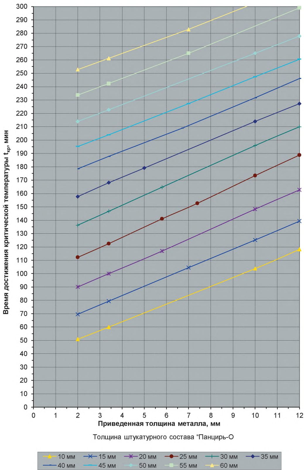
Рис. 22. Огнестойкость стальных конструкций с огнезащитным штукатурным составом "Панцирь О" при t_{кр} = 600\text{ }^{\circ}\text{C} .
