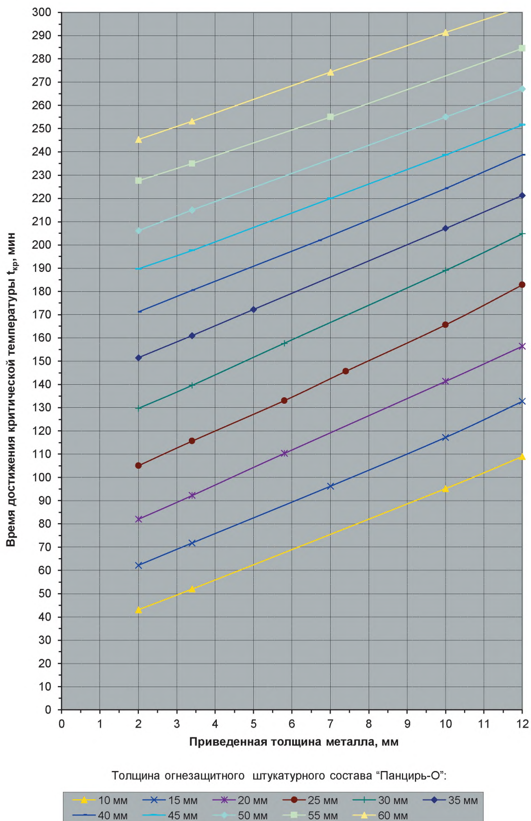
Рис. 21. Огнестойкость стальных конструкций с огнезащитным составом "Панцирь-О" при t_{кр} = 550^\circ\text{C} .
