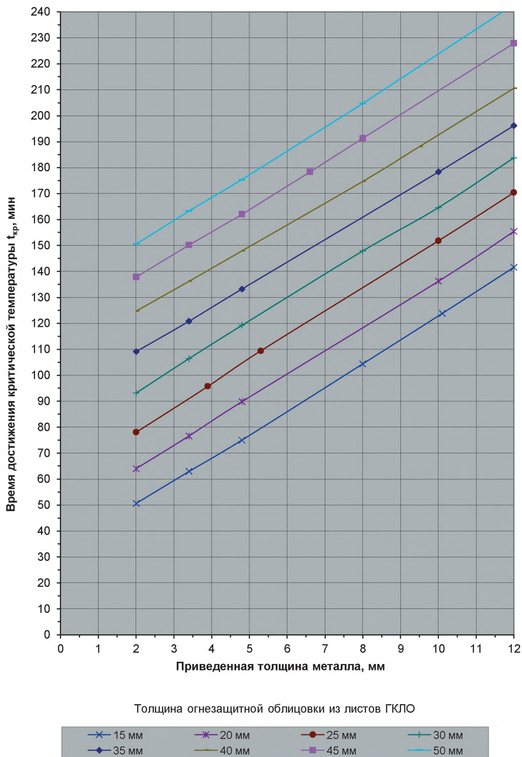
Рис. 13. Огнестойкость стальных конструкций с огнезащитной облицовкой из листов ГКЛО при t_{кр} = 550^\circ\text{C}
