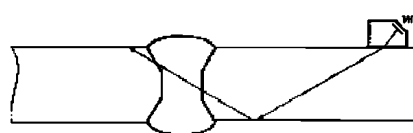
Б. Схема прозвучивания стыкового и углового сварного соединения однократно-отраженным лучом
