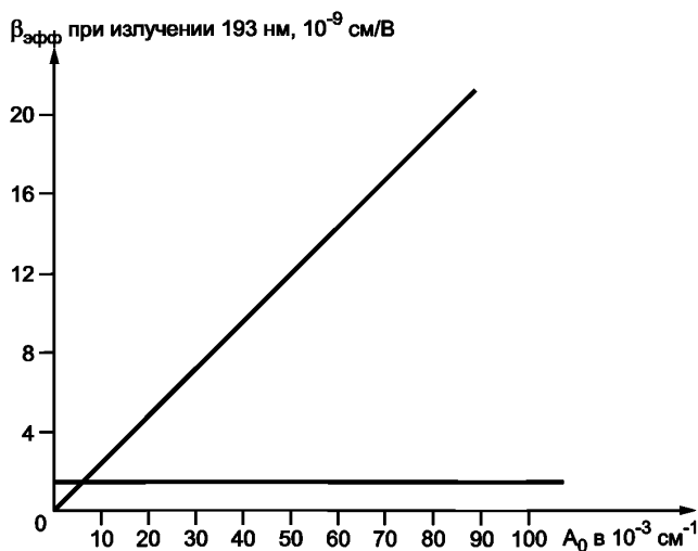
Рисунок 3 — Зависимости коэффициентов линейного и нелинейного поглощения для разных образцов \text{CaF}_2
