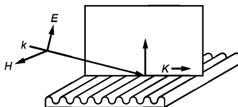
Рисунок 8 — p-поляризация
