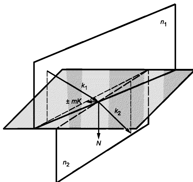
Рисунок 5 — Схематическое представление дифракции Рамана-Ната
