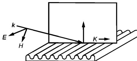
Рисунок 9 — s-поляризация
