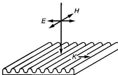
Рисунок 7 — ТМ-поляризация
