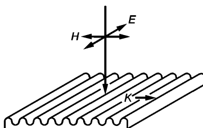
Рисунок 6 — ТЕ-поляризация
