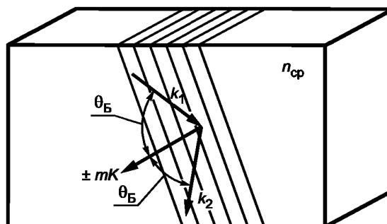
Рисунок 4 — Схематический чертёж дифракции Брэгга
