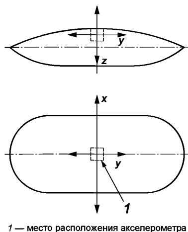
Рисунок 7 — Установка в адаптере трехкомпонентного акселерометра
