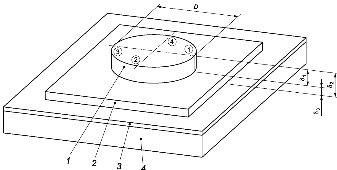
1 — измерительная масса; 2 — вибропоглощающий материал; 3 — лист из полиметилметакрилата; 4 — испытательный стол с плоской поверхностью; ①, ②, ③, ④ — точки измерений на верхней поверхности измерительной массы; D — диаметр измерительной массы; \delta_1 — высота измерительной массы; \delta_2 = \delta_1 + \delta_3 ; \delta_3 — толщина вибропоглощающего материала
