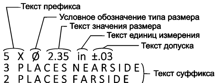
Рисунок 2 — Структурированная размерная надпись
