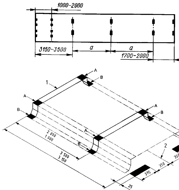
Рис. 2.3.2.5.2-4 Контактные площадки (контейнеры 1EEE, 1EE, 1AAA, 1AA, 1A и 1AX, имеющие паз «гусиная шея»): 1 — торец контейнера; 2 — центральная ось симметрии контейнера
