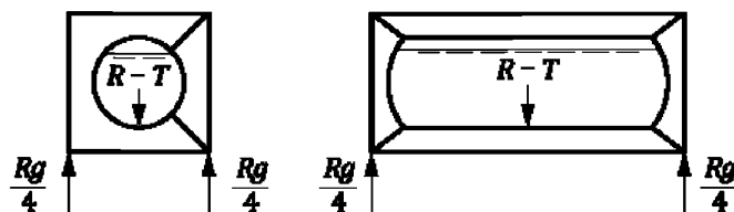
Рис. 3.4.1 Поперечное крепление
