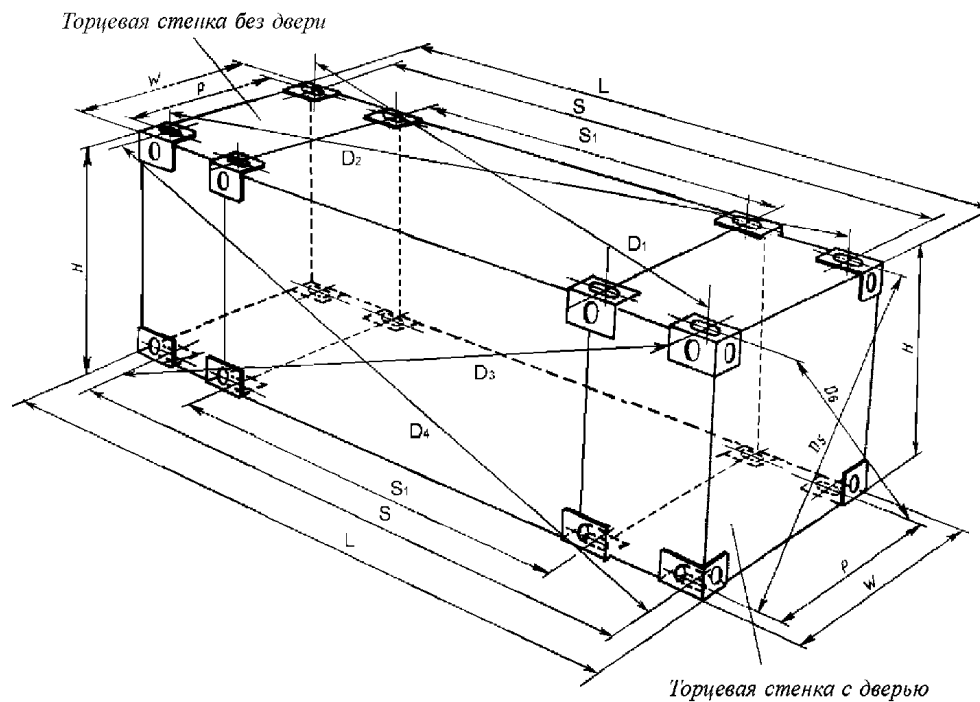
Рис. 2.2.1-6 Взаимное расположение фитингов в контейнерах IEEE, 1EE.
