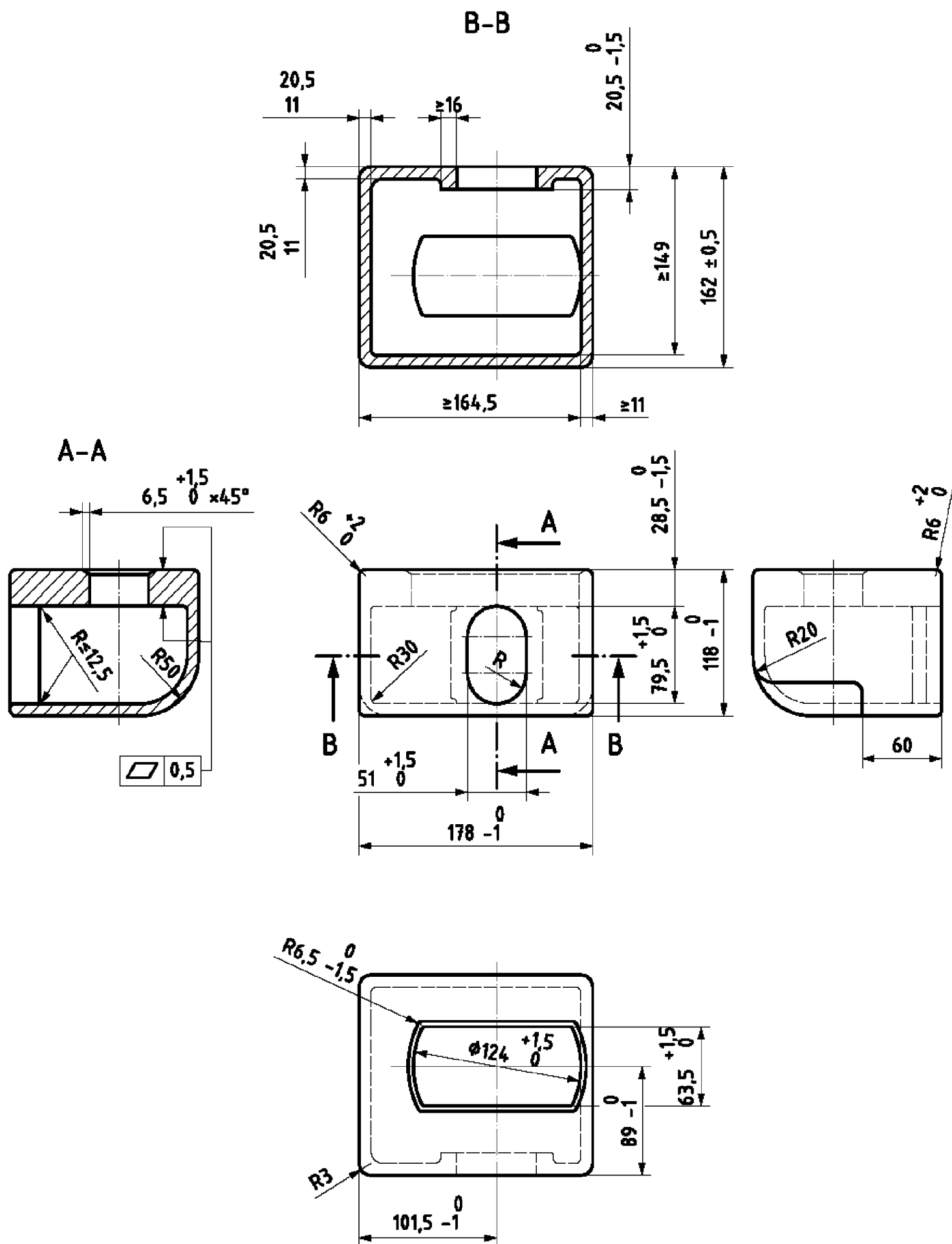
Рис. 2.2.1-3 Верхний промежуточный фитинг, мм
