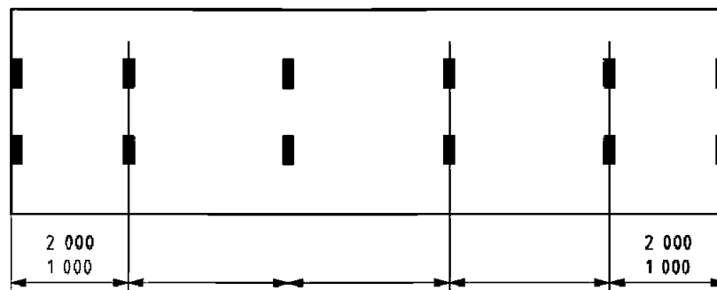
Рис. 2.3.2.5.1-2 Контактные площадки контейнеров 1BBV, 1BV, 1B, 1BX и 1CCS, имеющих 6 пар контактных площадок
