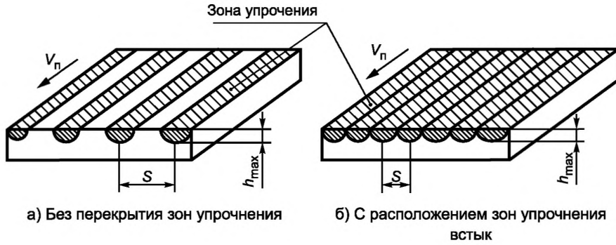
Рисунок 2 — Триботехнические рисунки лазерного термоупрочнения плоской поверхности
