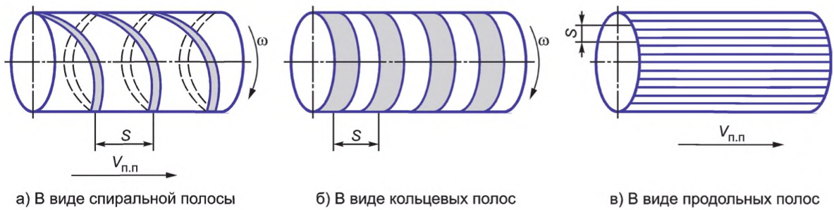
Рисунок 3 — Триботехнические рисунки лазерного термоупрочнения цилиндрической поверхности
