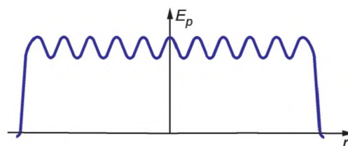
б) Распределение плотности мощности в пятне фокусировки
