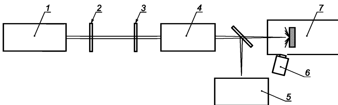
1 — лазерная система; 2 — переменный аттенюатор; 3 — фазовая пластинка; 4 — фокусирующая система; 5 — блок диагностики пучка; 6 — система онлайн-обнаружения разрушения; 7 — отсек для образцов
