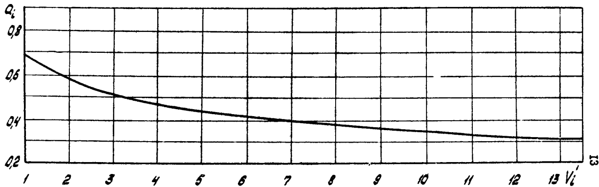
Рис.3. Зависимость a_i = 1 - \left(\frac{\mu a_i}{\mu_i}\right)^{\alpha_i' (1 - a_i)} от относительной скорости струи V_i'
