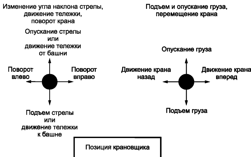
Рисунок 1 — Схема расположения основных органов управления башенным краном
