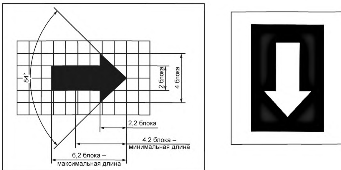
Рисунок Г.22 — Стрелка для отображения направления давления или усилия
