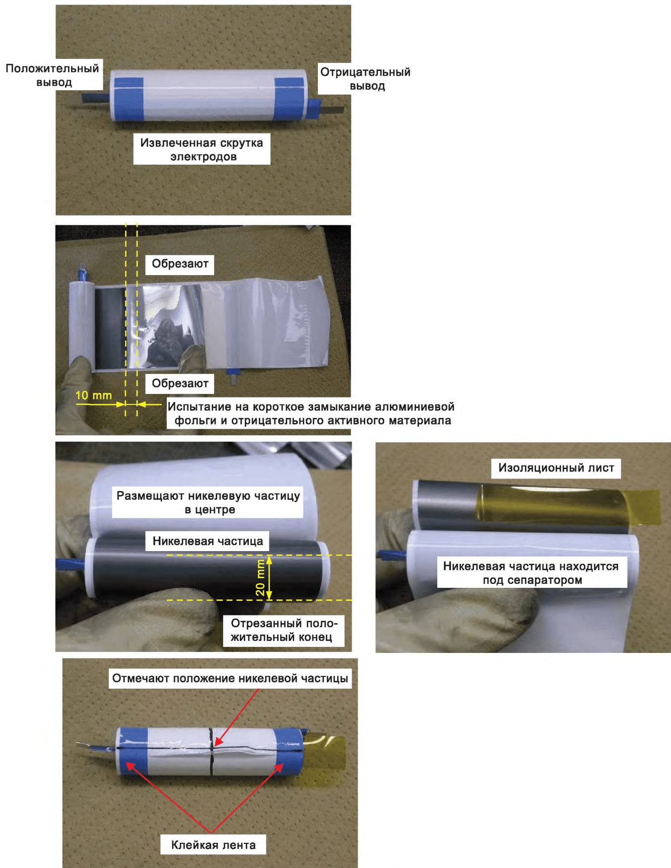
Рисунок А.6 — Разборка цилиндрического аккумулятора
