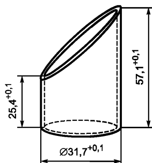
Рисунок 7 — Шаблон проглатывания
