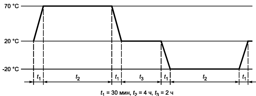
Рисунок 2 — Температурный цикл
