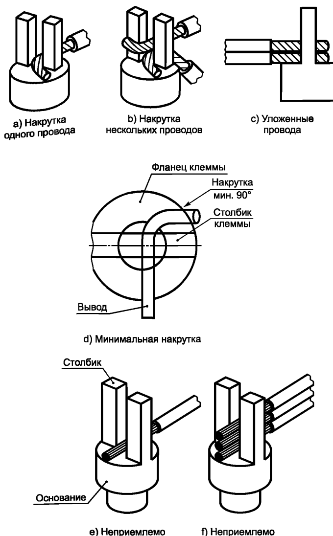
Рисунок 6 — Монтаж в разрезной контакт
