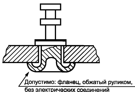
Рисунок 1 — Контакт с развальцованным фланцем
