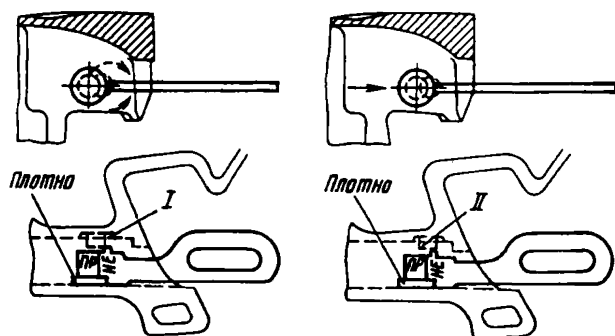
Рис. 2.13. Проверка высоты шипа для замкодержателя шаблоном 849р-1:
