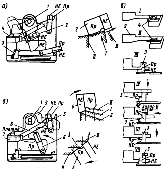
Рис. 2.30. Проверка противовеса, расцепного угла и отверстия замкодержателя шаблоном 826p
