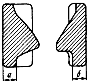
Рис. 2.45. Фрикционные клинья поглощающих аппаратов
