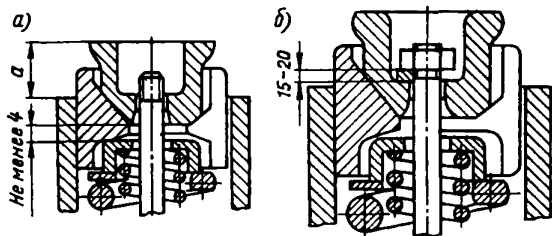
Рис. 2.47. Положение нажимного конуса в собранном поглощающем аппарате до постановки гайки стяжного болта ( a ) и размещение подкладки под гайкой стяжного болта поглощающего аппарата ( b )
