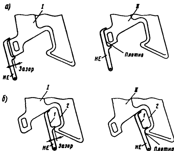
Рис. 2.2. Проверка шаблонами 892р, 893р, 884р:
