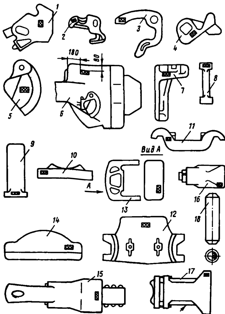
Рис. 2.61. Детали автосцепного устройства (заштрихованы места расположения клейм):
