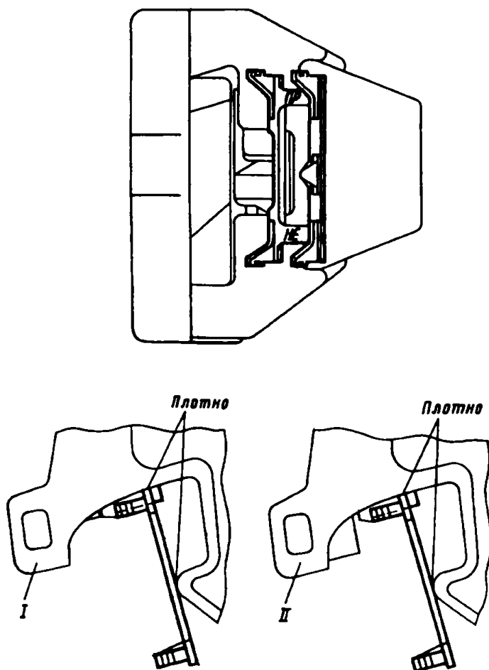
Рис. 2.38. Проверка шаблоном 820р надежности удержания замка в расцепленном состоянии при выходе лапы замкодержателя в зев на 25 мм
