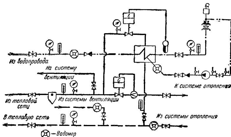
Рис. 8. Схема установки водометров для учета тепла на тепловом пункте в закрытой водяной тепловой сети.
