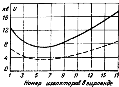
Рис. 6. Распределение напряжения по гирлянде из 17 изоляторов марки П-4,5 на ВЛ 330 кв.
