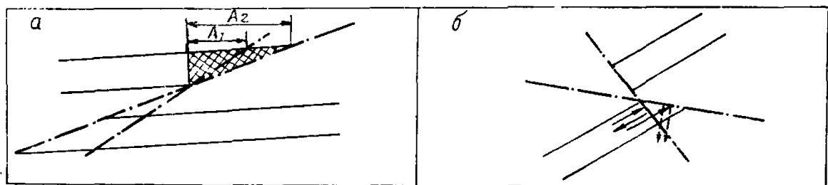
Рис. 9. Характер изменения величины потерь ( a ) и отражения сейсмических волн ( б ) при согласном и несогласном залегании пласта и сместителя:
