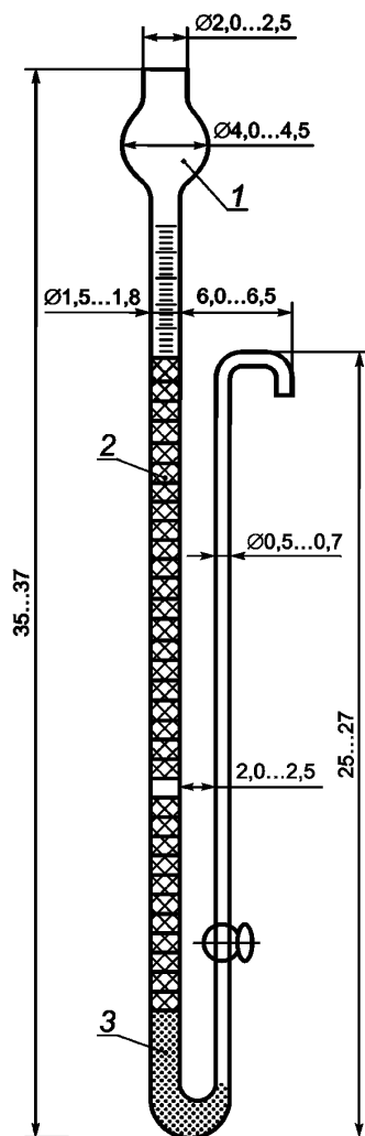
1 — анализируемый раствор; 2 — катионитовая смола; 3 — стеклянная вата
