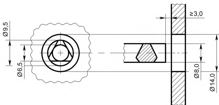
Рисунок Б.1 — Ключевина устройства отпирания замка
