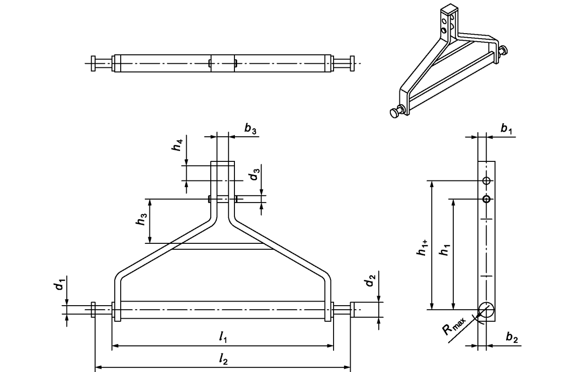
а) С консольно установленными пальцами
