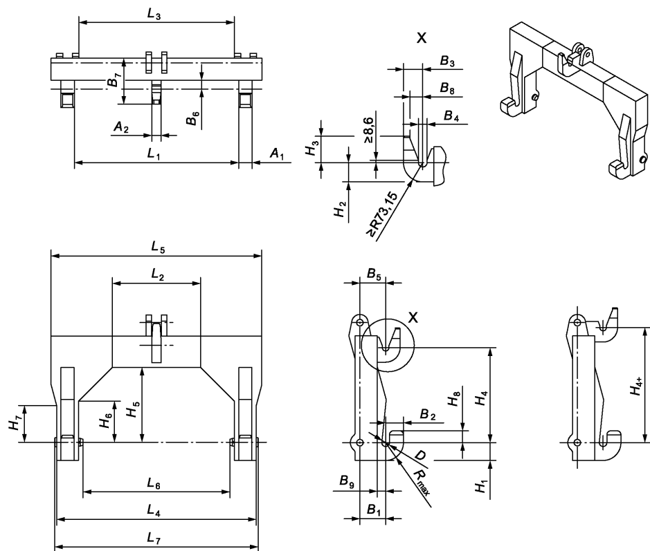
Рисунок 1 — Размеры сцепного устройства
