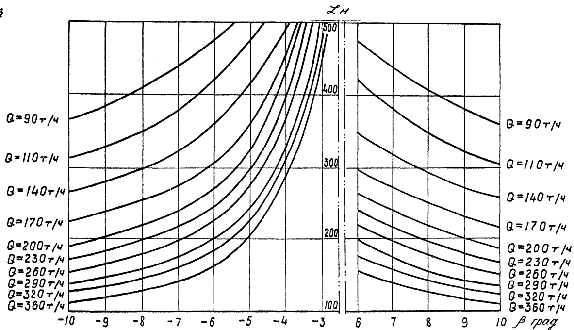
Рис. 2. Зависимость длины конвейера KL-I50V2 от угла наклона и производительности
