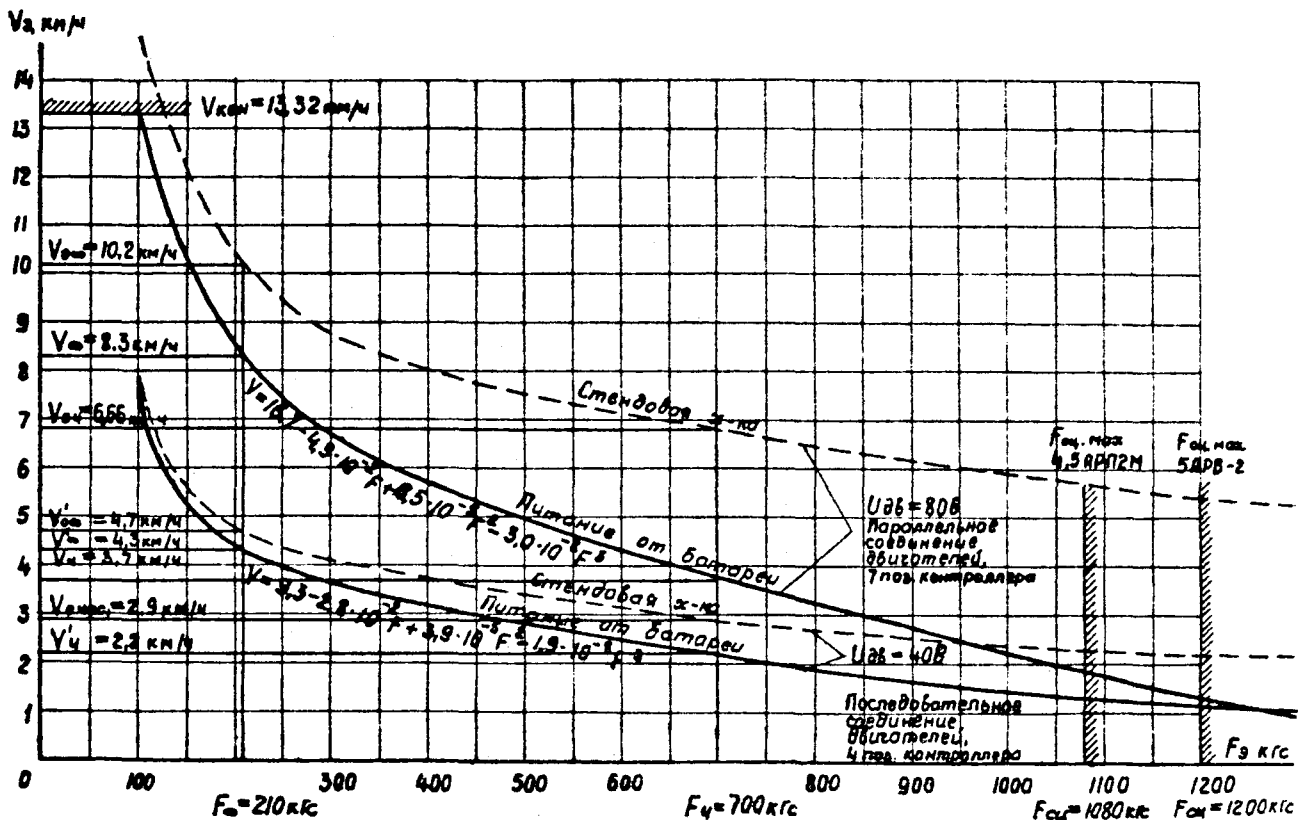
Рис. 2. Типовые характеристики рудничных аккумуляторных электровзозов 5АРВ-2 и 4,5АРВ-2М с аккумуляторными батареями 66ТЭН-250П и 66ТЭН-300 и электродвигателем ЭДР-7П
