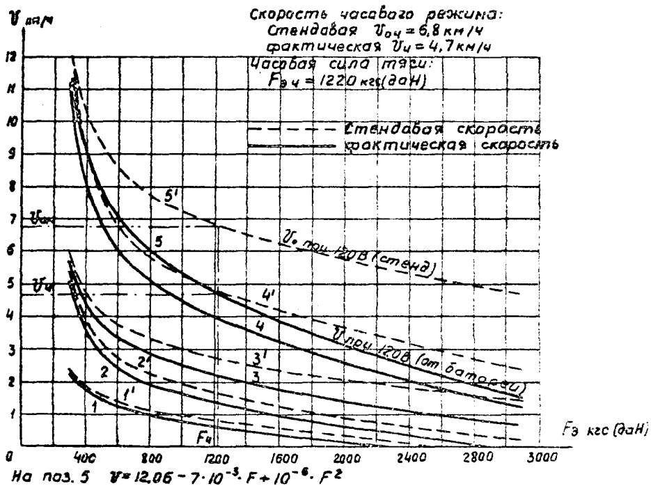
Рис. 8. Тяговые характеристики рудничного аккумуляторного электровоза АМВД на колесах 600 мм с аккумуляторной батареей 96ТДН-350 и электродвигателем ДЭР-12
