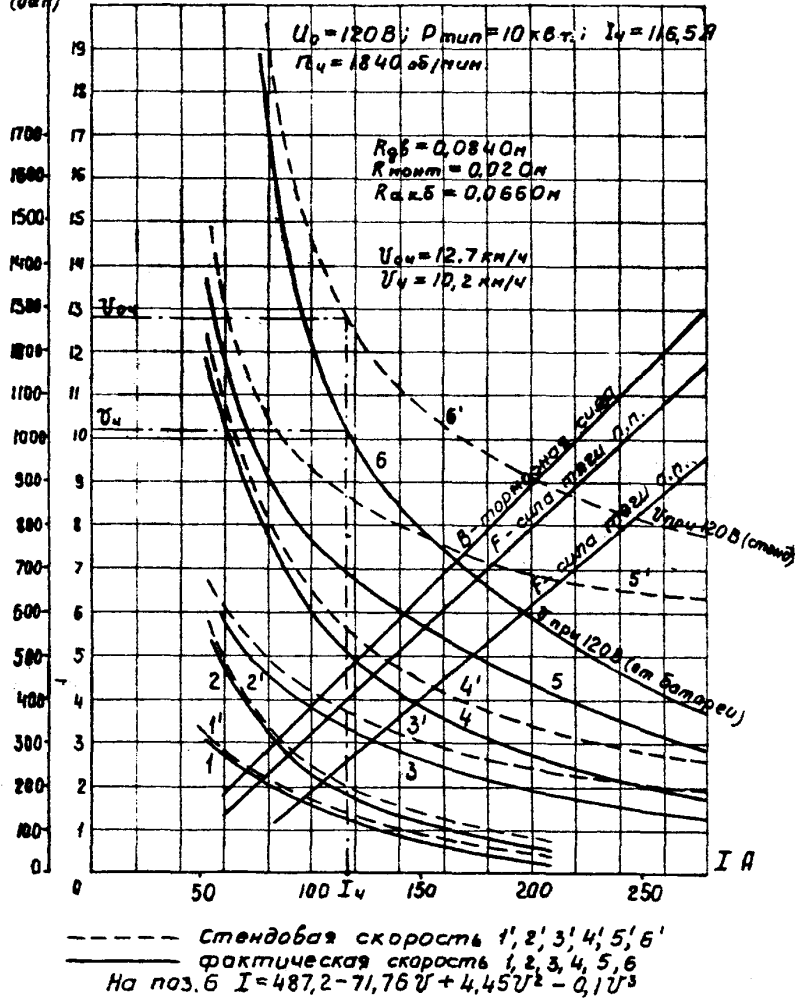
Рис. II. Характеристики электродвигателя ДРТ-10, приведенные к ободу колеса электровоза АРП7-900 (АРВ7-900) с аккумуляторной батареей ГСЭТНМ-550
