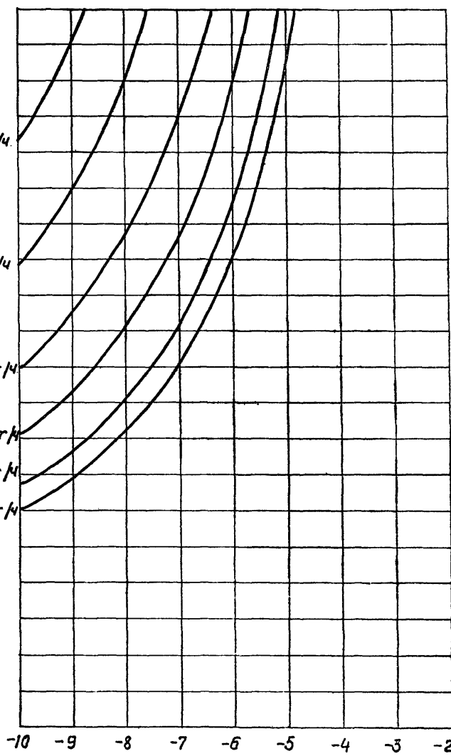
Рис. 19. Зависимость длины конвейера ЛНТ100 от угла наклона и производительности при V = 1,6 \text{ м/с} и \rho = 200 \text{ кВт}
