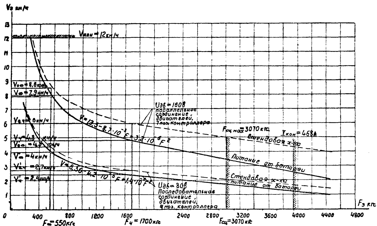
Рис. 7. Тяговые характеристики рудничного аккумуляторного электровоза IЗАР-I с аккумуляторной батареей I26ТДН-550 и электродвигателем ЭДР-15
