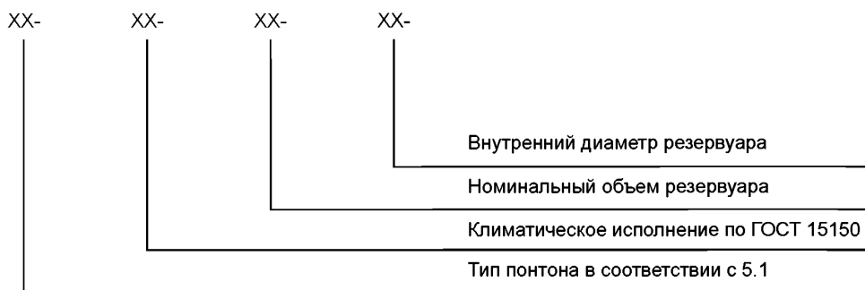
Рисунок 1 — Схема условного обозначения понтона
