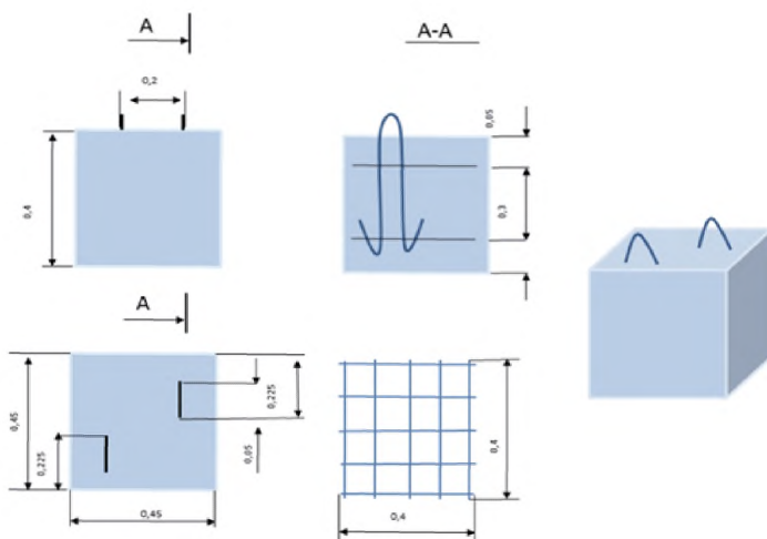
Рисунок 1 – Железобетонная тумба
