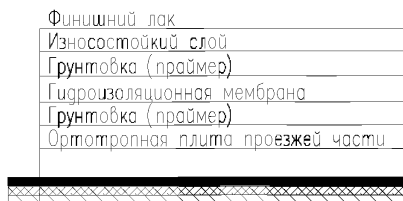
Рисунок 5.3 – Вариант конструкции тонкослойного полимерного покрытия на основе ПММА на ортотропной плите проезжей части моста
