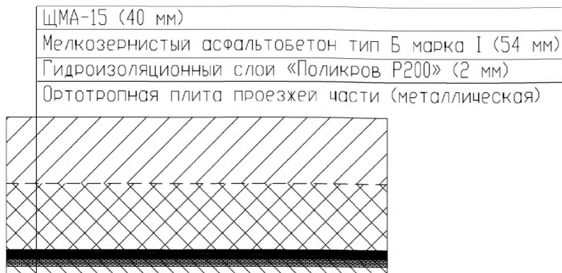
Рисунок А.8 – Конструкция одежды ездового полотна на мосту через пролив Босфор Восточный в г. Владивостоке
