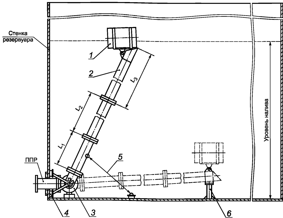
Рисунок А.5 — Общий вид приемо-раздаточного устройства специального типа с плавающим заборным устройством
