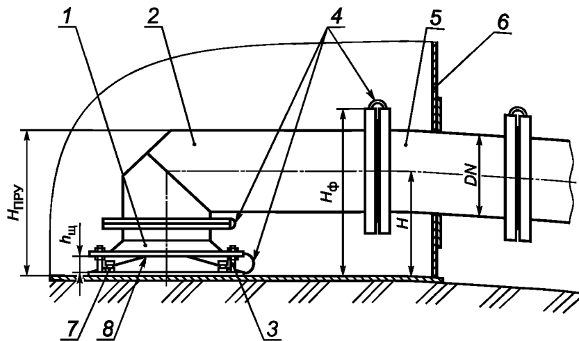
а) При высоком расположении приемо-раздаточного патрубка ( H_{\text{ПРУ}} < H_{\text{Ф}} )
