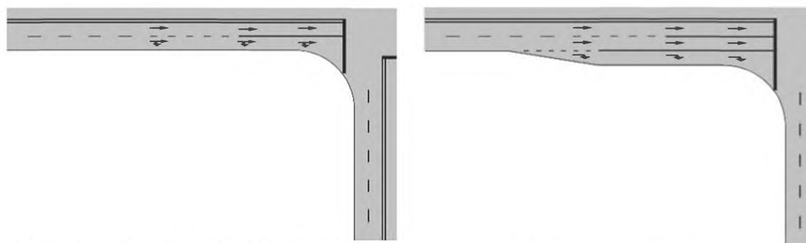
б) Полоса для поворота без направляющего островка
