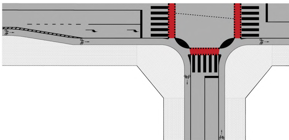
Рисунок 22 — Пример расположения велосипедной полосы относительно полосы для поворота направо
