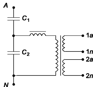
Рисунок 503 — EHN с двумя вторичными обмотками
