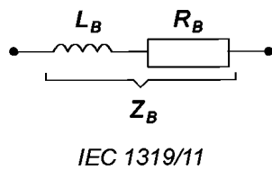
Рисунок 510 — Последовательная нагрузка
