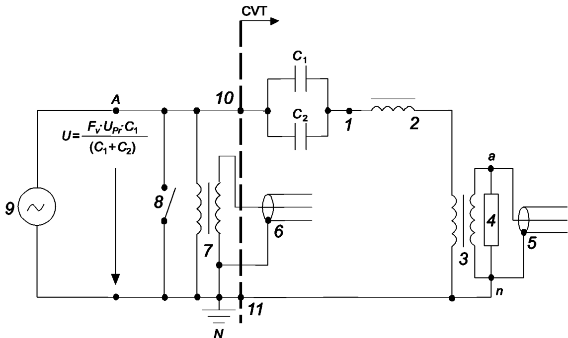
1 — вывод промежуточного напряжения; 2 — компенсационная индуктивность; 3 — трансформатор промежуточного напряжения; 4 — нагрузка Z_B ; 5 — запись напряжения вторичной обмотки; 6 — запись напряжения первичной обмотки; 7 — измерительный трансформатор напряжения; 8 — устройство для создания короткого замыкания; 9 — источник напряжения; 10 — выводы высокого напряжения; 11 — выводы заземления
