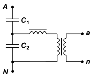
Рисунок 502 — EHN с одной вторичной обмоткой
