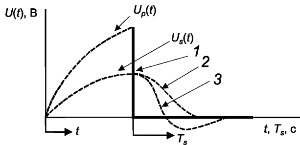
1 — короткое замыкание U_P(t) ; 2 — апериодическое демпфирование U_S(t) ; 3 — периодическое демпфирование U_S(t)
