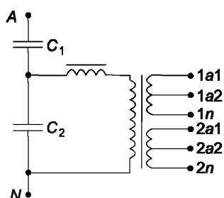
Рисунок 504 — EHN с двумя секционированными вторичными обмотками
