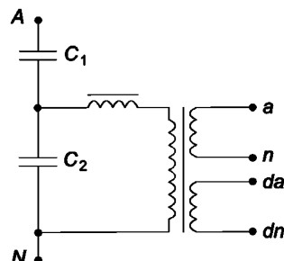
Рисунок 505 — EHN с одной обмоткой напряжения нулевой последовательности и одной вторичной обмоткой
