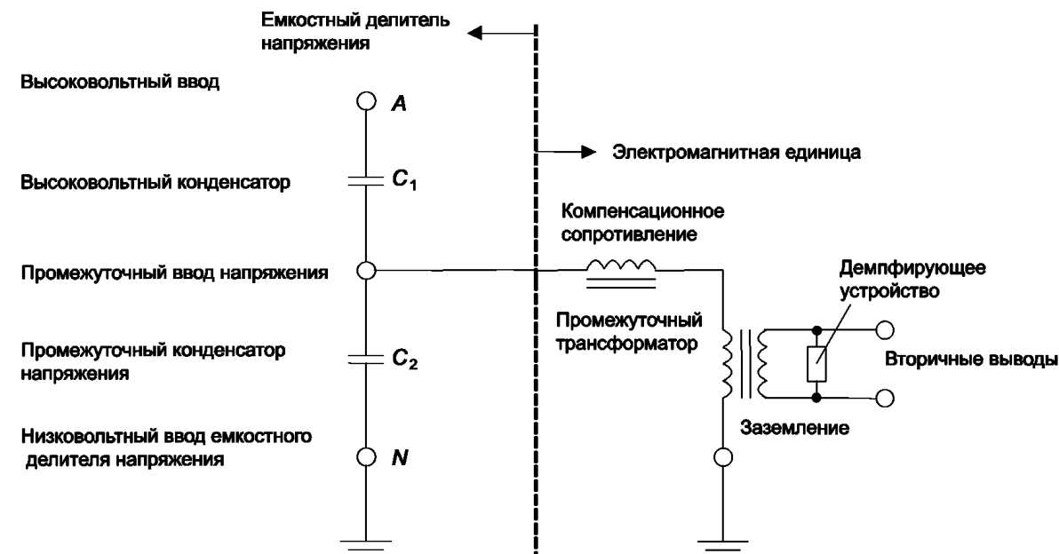
Рисунок 5А.1 — Пример диаграммы для емкостного трансформатора напряжения
