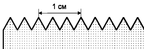
Рисунок 1 — Поглощающая мишень в разрезе
