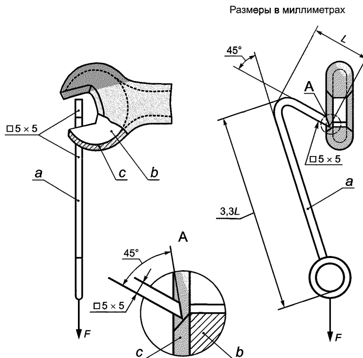
a — крюк (длина плеча зависит от размера инструмента); b — токоведущая часть с покрытием из изоляционного материала; L — длина короткого плеча крюка
