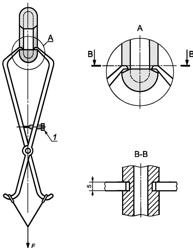
1 — регулировочное устройство
