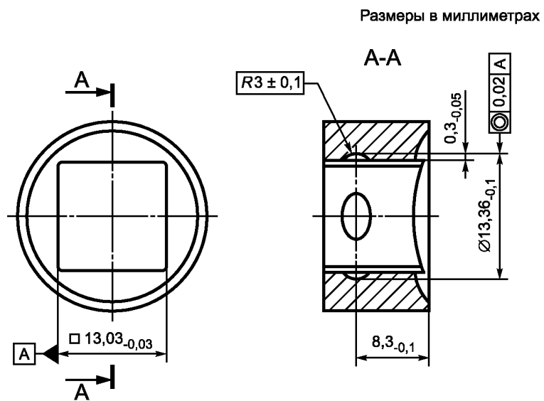
Рисунок 25 — Имитатор для испытания систем блокировки, используемых в инструментах с соединительным квадратом номинальным размером 12,5 мм ISO 1174-1
