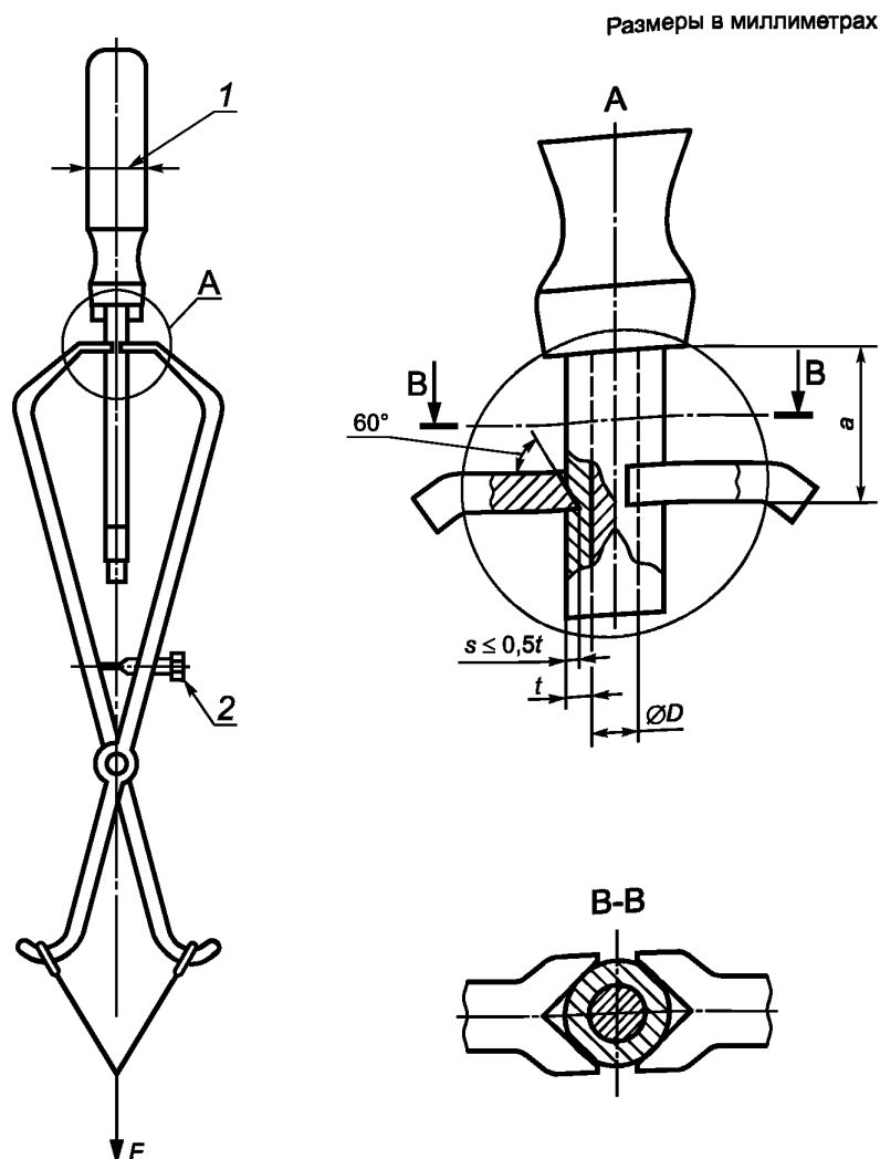
1 — зажимное устройство для фиксации отвертки во время испытания вертикально, стержнем вниз; 2 — регулировочное устройство; s — глубина проникновения ( s \leq 0,5t ); t — толщина покрытия изоляционного материала; F — испытательная сила; a — расстояние от 10 до 15 мм между точкой, в которой стержень выходит из рукоятки и режущей кромкой испытательного прибора; D — диаметр стержня
