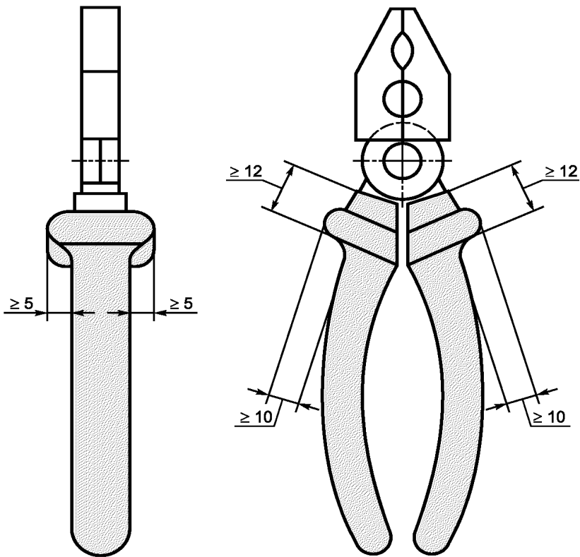
Рисунок 8 — Изоляция плоскогубцев
