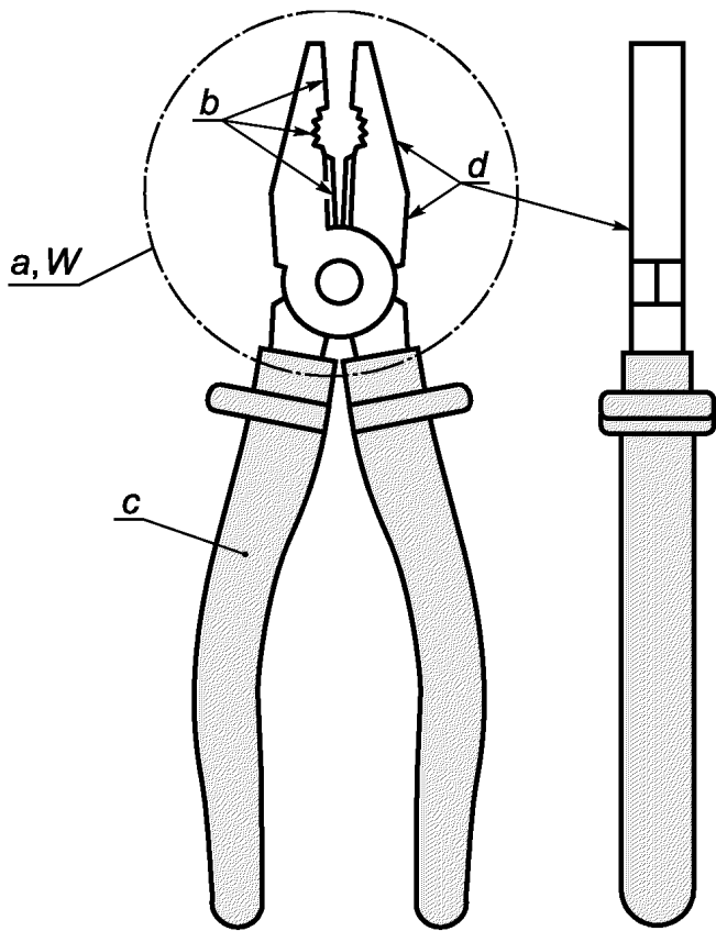
a — токоведущая часть; b — рабочая поверхность; c — изоляция; d — область контакта; W — рабочая головка
