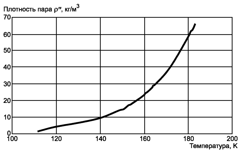
Рисунок А.3 — Плотность насыщенного пара метана
