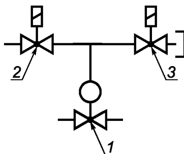
1 — исполнительный механизм при испытаниях; 2 — пилотный клапан (полностью закрытый); 3 — выпускной клапан (полностью открытый)
