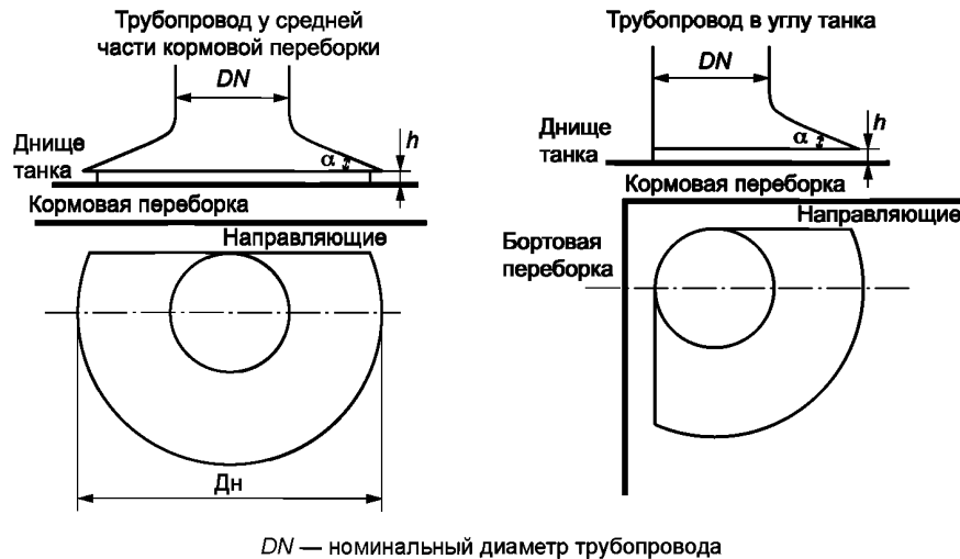
Рисунок Б.1 — Конструкция антистатического патрубка
