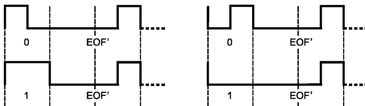
Рисунок 28 — Метод ASK: символ EOF, завершающий FM0 передачу
