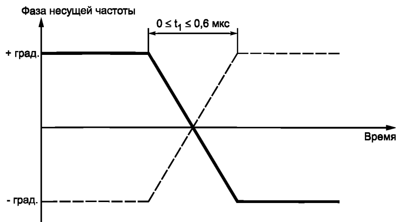
Рисунок 20 — Метод PJM: схема модуляции команд
