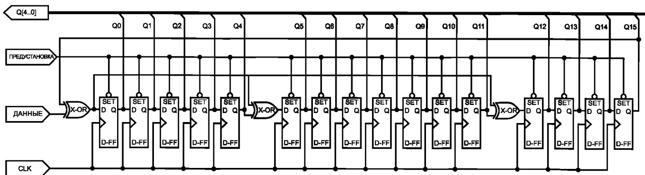
Рисунок 1.2 — Пример схемы кодека CRC-16с
