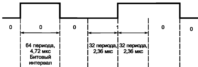
Рисунок 18 — Метод P1M: MFM кодирование команды и временные диаграммы двоичной последовательности 000100
