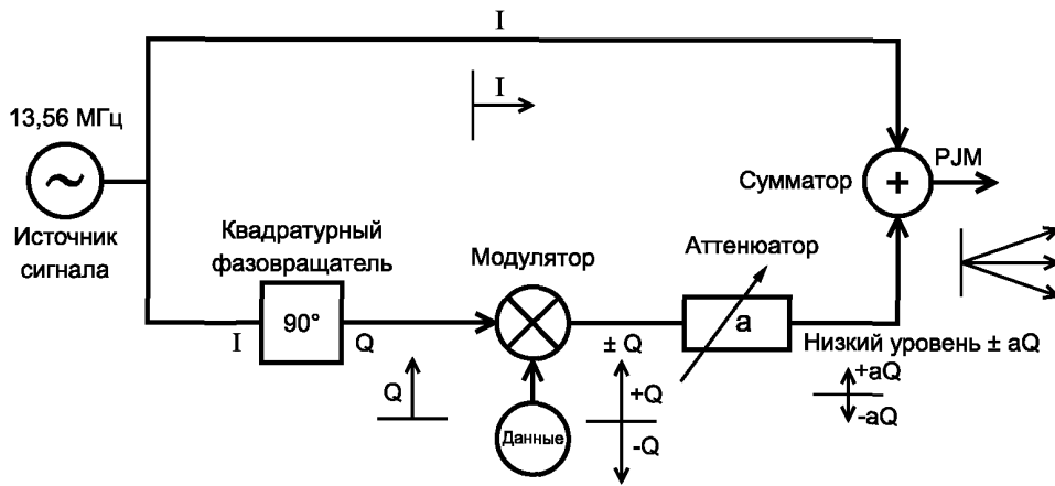
Рисунок В.5 — Пример реализации — цепь для генерации PJM, показывающая различные элементы сигнала PJM
