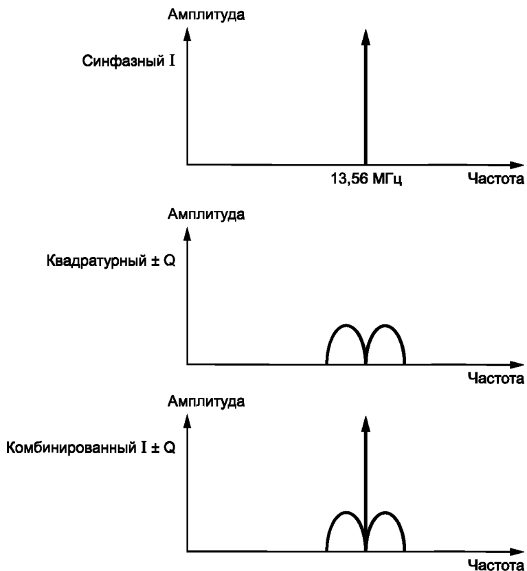
Рисунок В.3 — Формирование PPM
