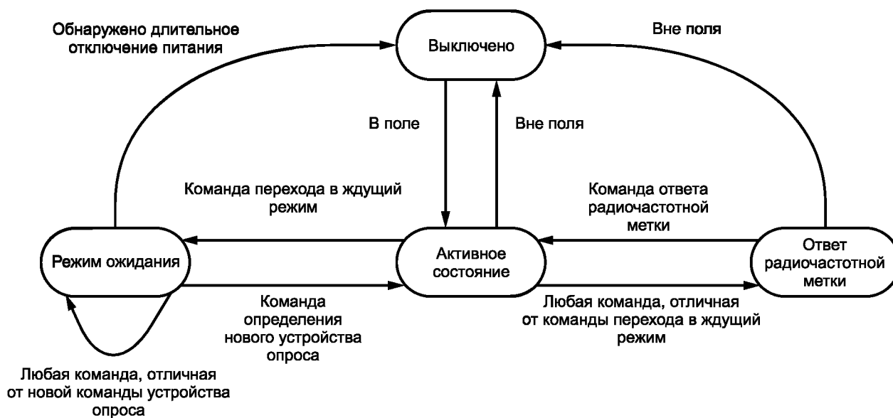
Рисунок 10 — Диаграмма изменений состояния радиочастотной метки
