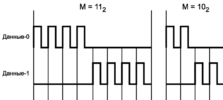
Рисунок 30 — Метод ASK: Манчестерское кодирование последовательности на поднесущей
