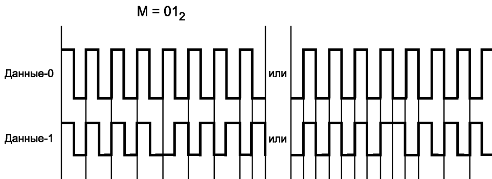
Рисунок 34 — Метод ASK: Последовательность кода Миллера на поднесущей
