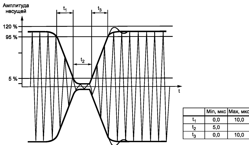
Рисунок 11 — Отключение силового питающего поля УСО
