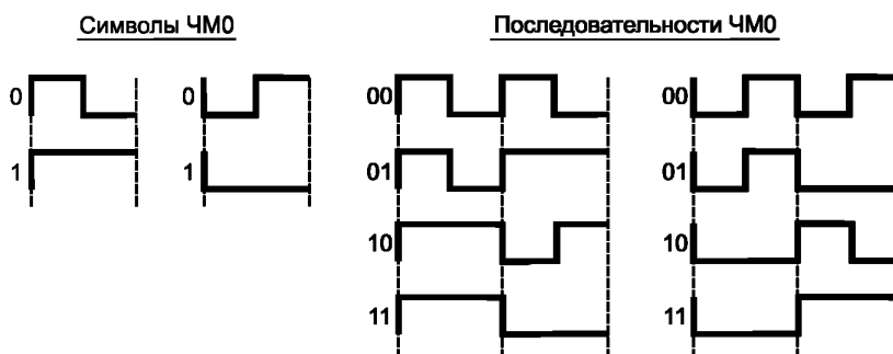
Рисунок 26 — Метод ASK: FM0 символы и последовательности
