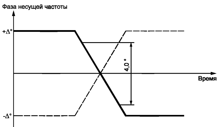
Рисунок 3 — Схема модуляции команды
