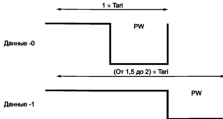
Рисунок 17 — Метод ASK: символы P1E
