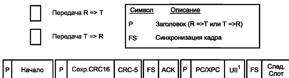
Рисунок 45 — Ответ одной радиочастотной метки
