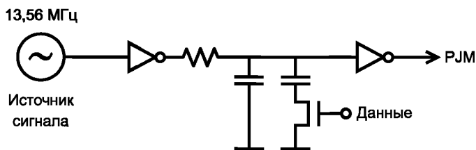
Рисунок В.4 — Пример реализации — простая цепь для обеспечения управляемого данными переменного сдвига фазы для генерации PPM
