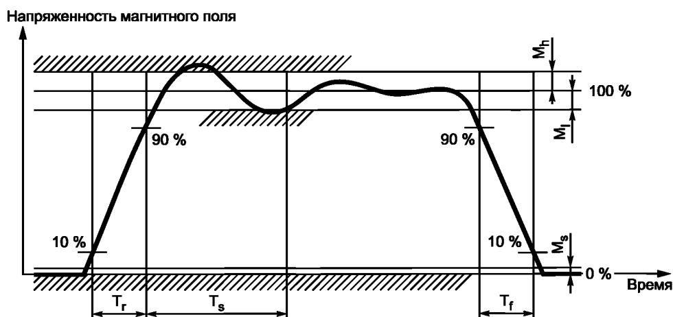
Рисунок 21 — РЧ огибающая включения и выключения питания УСО
