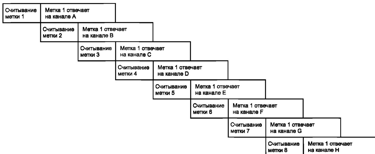
Рисунок 13 — Считывание данных из 8 радиочастотных меток
