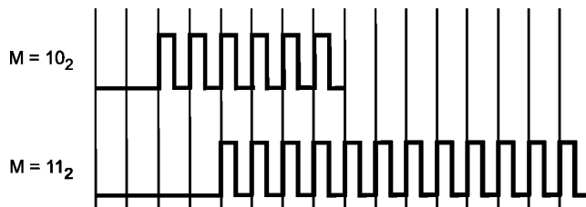
Рисунок 32 — Метод ASK: Символ EOF завершающий передачу поднесущей
