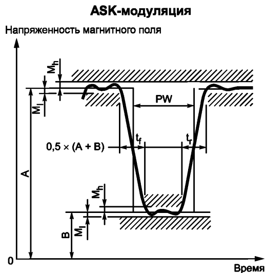
Рисунок 19 — Метод ASK: Огибающая сигнала «УСО-радиочастотная метка»
