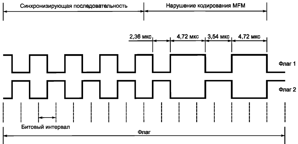
Рисунок 5 — MFM кодирование и временные диаграммы для двух возможных флагов команды
