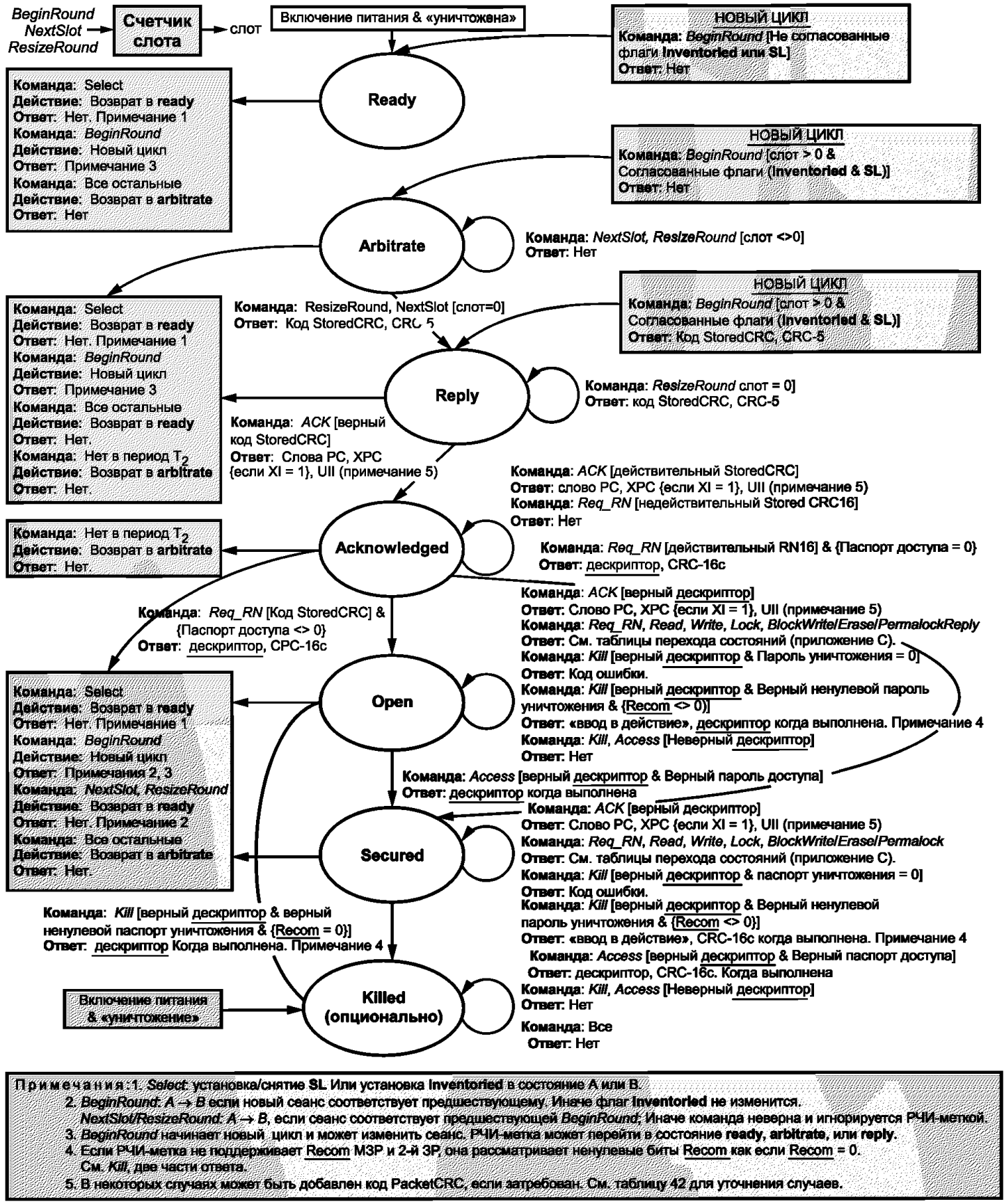
Рисунок 43 — Диаграмма состояний радиочастотной метки
