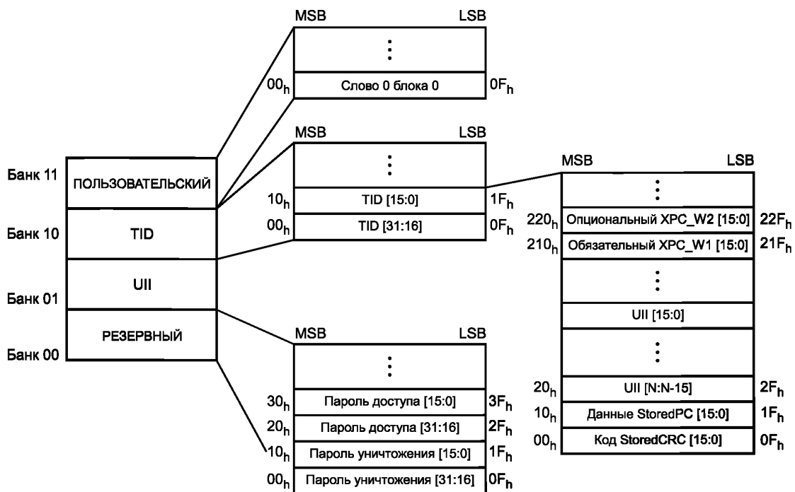
Рисунок 41 — Карта распределения памяти
