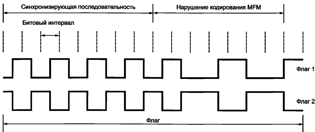
Рисунок 1 — Два возможных флага команд
