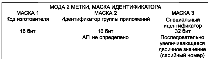
Рисунок 9 — Логическая организация идентификатора радиочастотной метки
