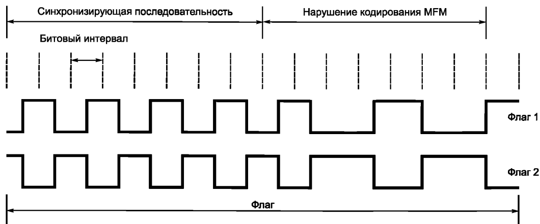
Рисунок 2 — Два возможных флага ответа
