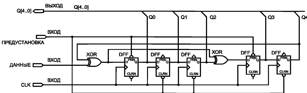
Риснок I.2 — Пример схемы кодека CRC-5
