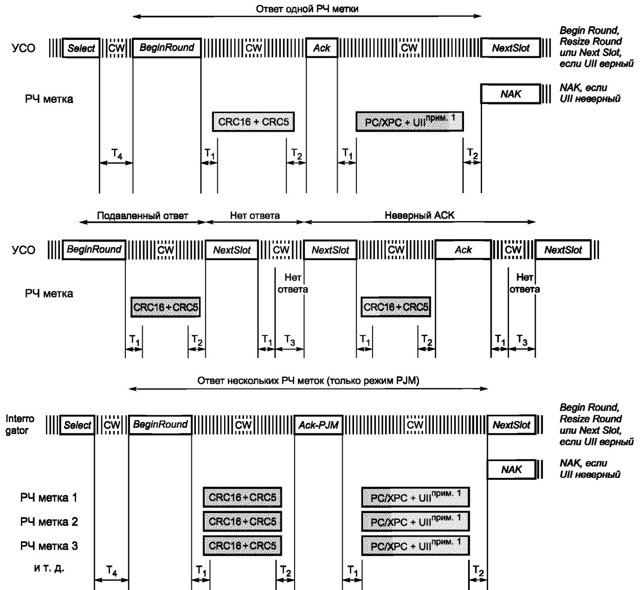
Рисунок 40 — Временные диаграммы синхронизации соединения — оба метода
