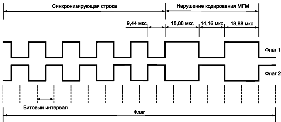
Рисунок 39 — Метод PJM: Флаги поднесущей T=>R
