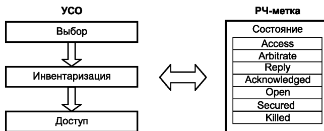
Рисунок 44 — Операции УСО/радиочастотной метки и состояния радиочастотной метки
