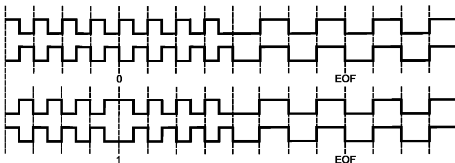
Рисунок 36 — Метод ASK: Символ EOF, завершающий передачу поднесущей
