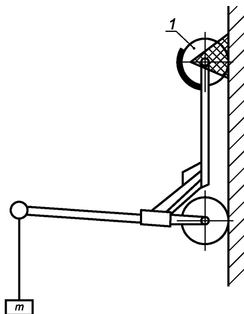
1 — фиксация заднего колеса (самокат может свободно вращаться)
