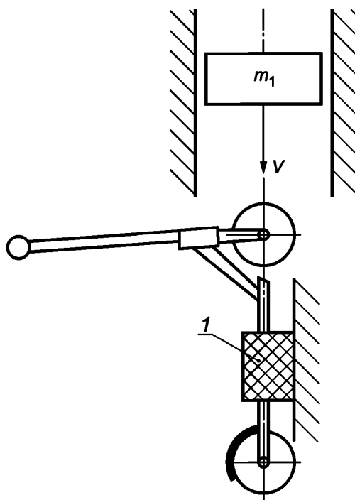
1 — фиксатор образца
