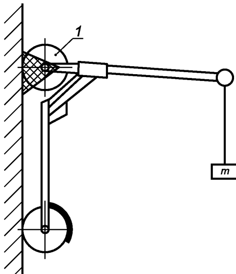
1 — фиксация переднего колеса (самокат может свободно вращаться)
