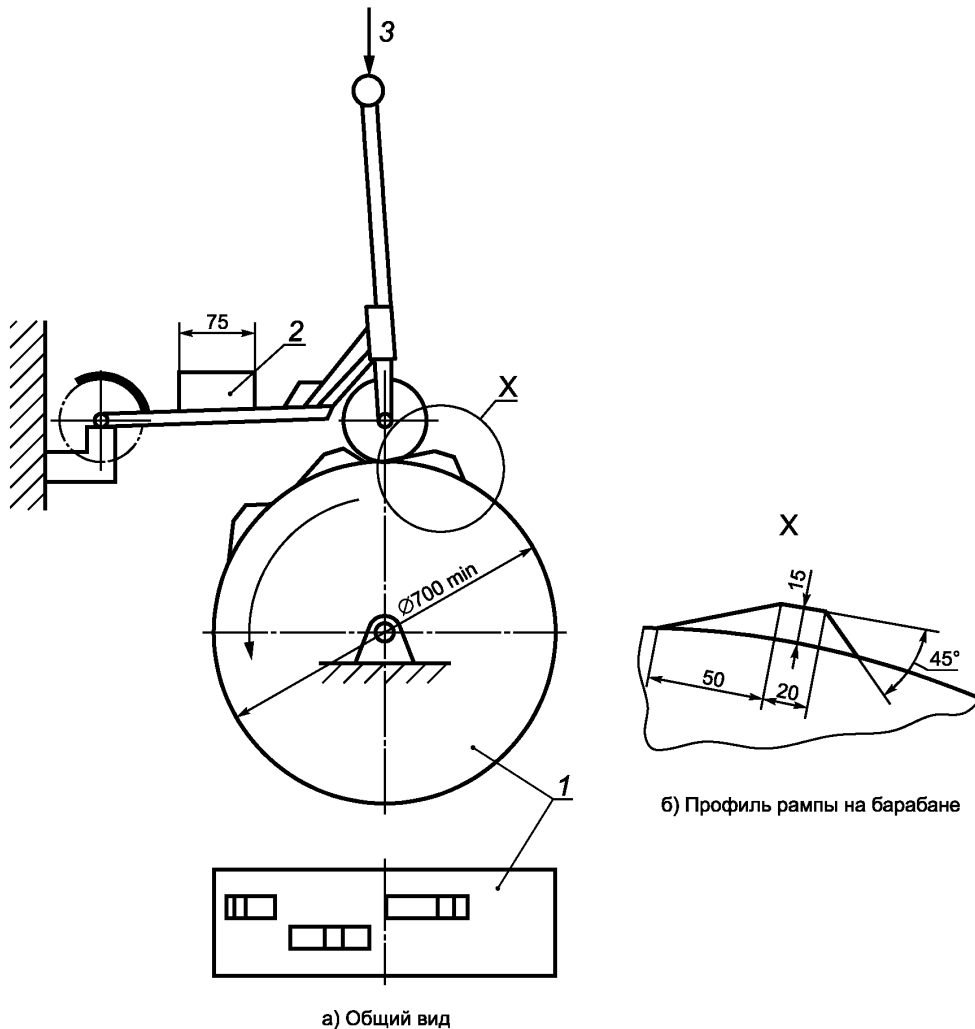
1 — барабан; 2 — масса: 90 кг для класса А и 45 кг для класса В; 3 — масса: 10 кг для класса А и 5 кг для класса В
