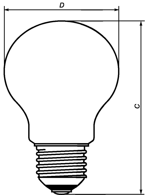
Рисунок 2 — Лампа с резьбовым цоколем Эдисона
