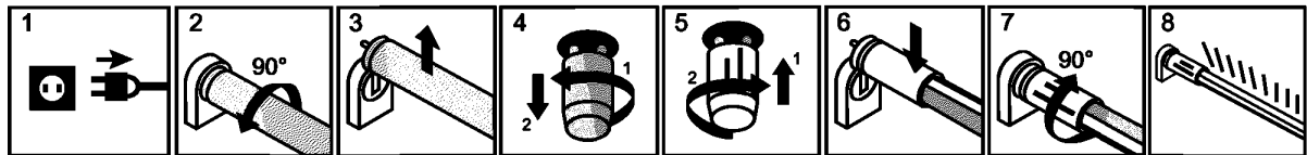
Рисунок 7 — Схематические этапы извлечения люминесцентной лампы и вставки двухцокольной СД-лампы, предназначенной для замены линейной люминесцентной лампы
