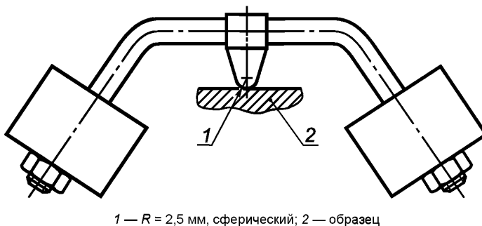
Рисунок 10 — Устройство для испытания давлением шарика
