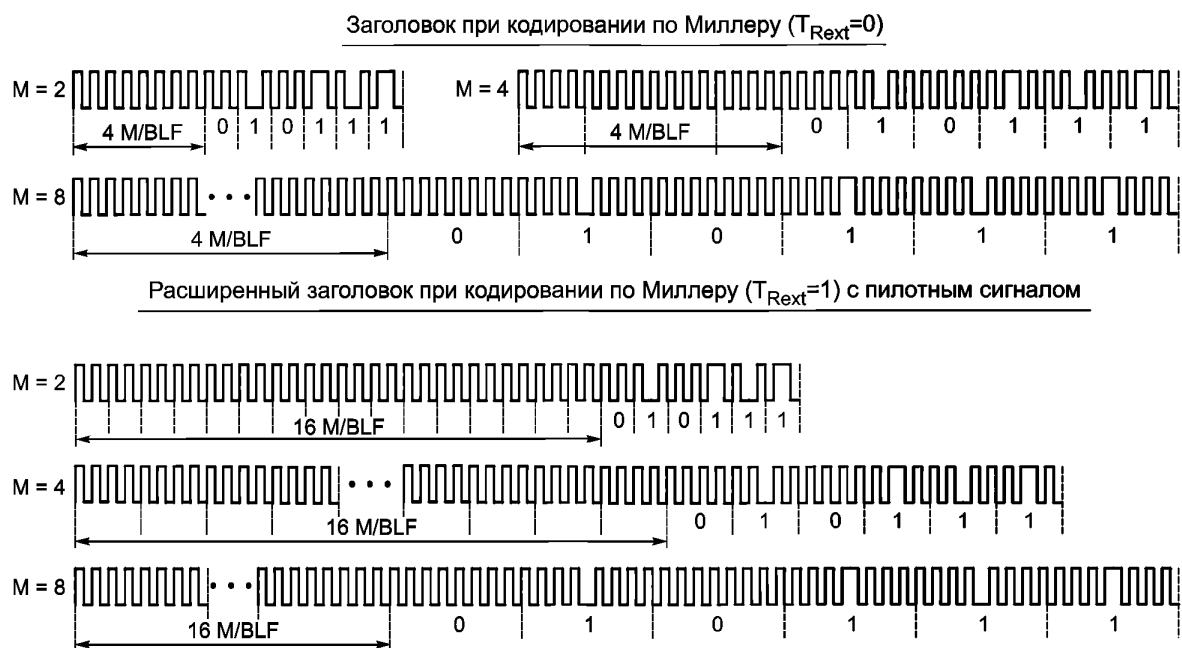
Рисунок 6.15 — Заголовок сигнала поднесущей в линии связи T \Rightarrow R
