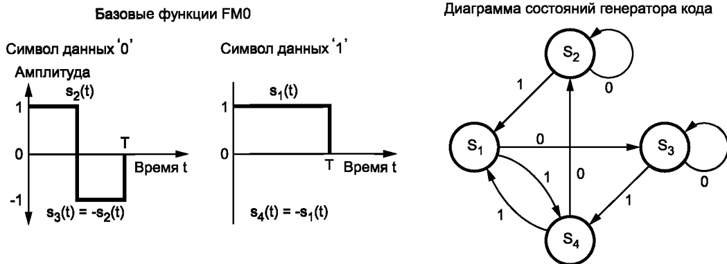
Рисунок 6.8 — Базовые функции FM0 и диаграмма состояний генератора кода
