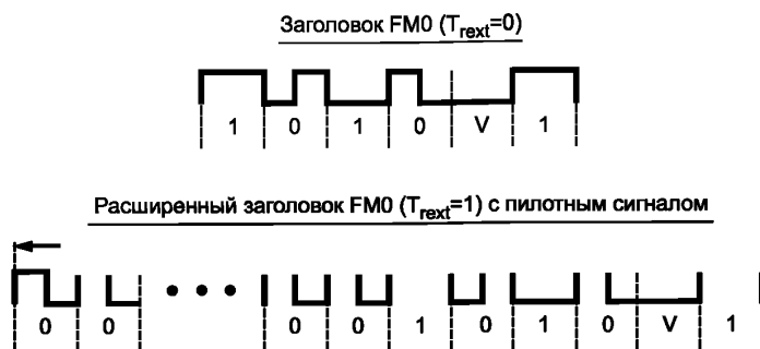
Рисунок 6.11 — Заголовок, закодированный методом FM0, для передачи по линии связи T \Rightarrow R
