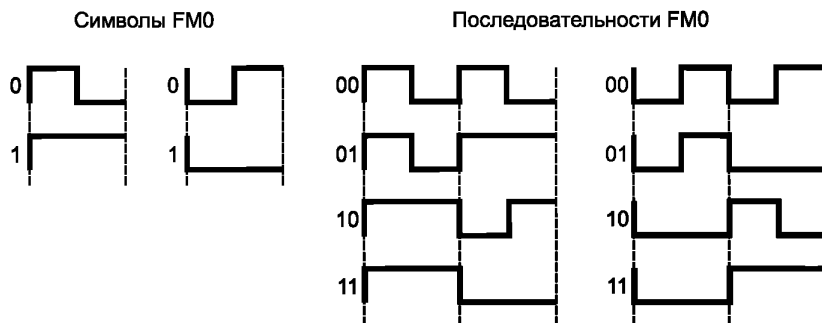
Рисунок 6.9 — Символы и последовательности, закодированные методом FM0
