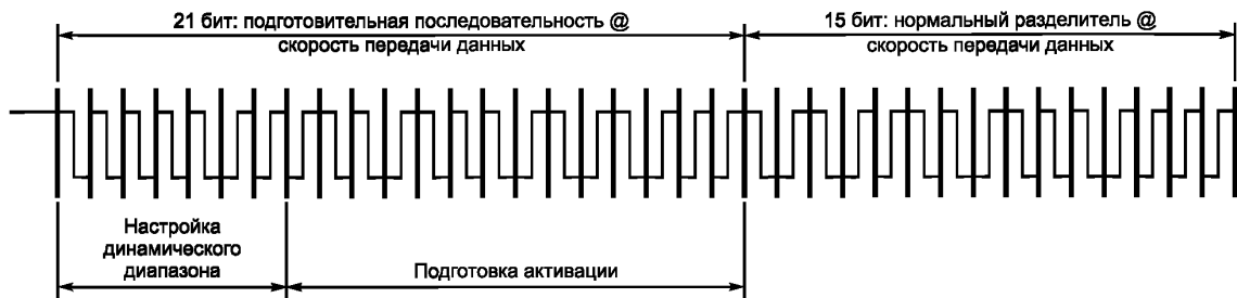
Рисунок 7.4 — Заголовок прямой линии связи (R=&gt;T)
