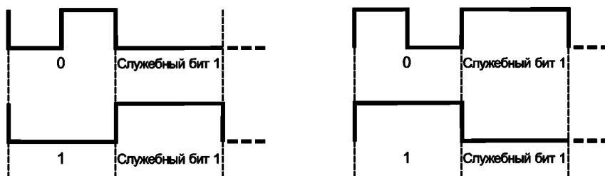
Рисунок 6.10 — Окончание передачи FM0
