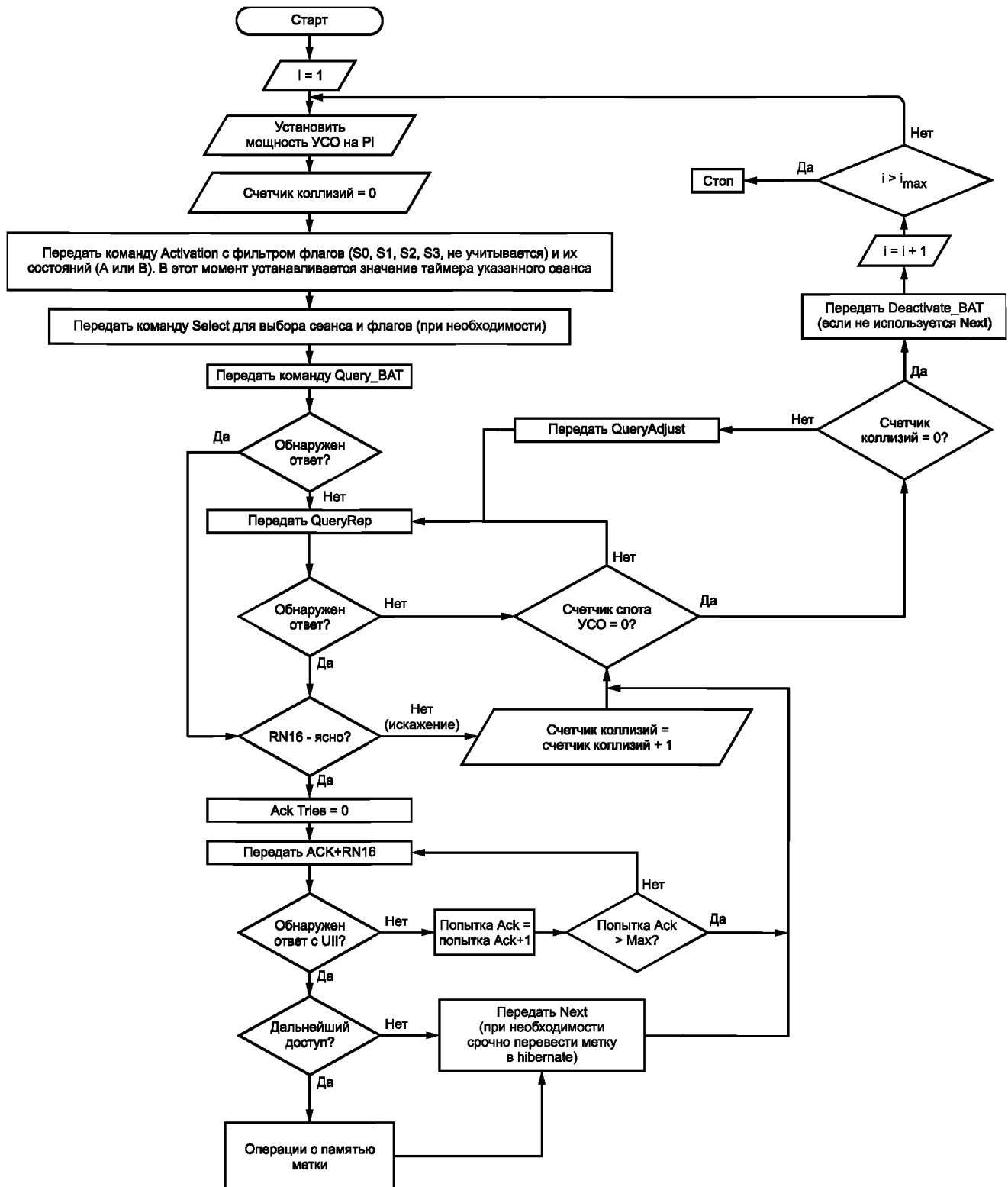
Рисунок R.2 — Типичная блок-схема процесса управления мощностью (функция Power Levelling)
