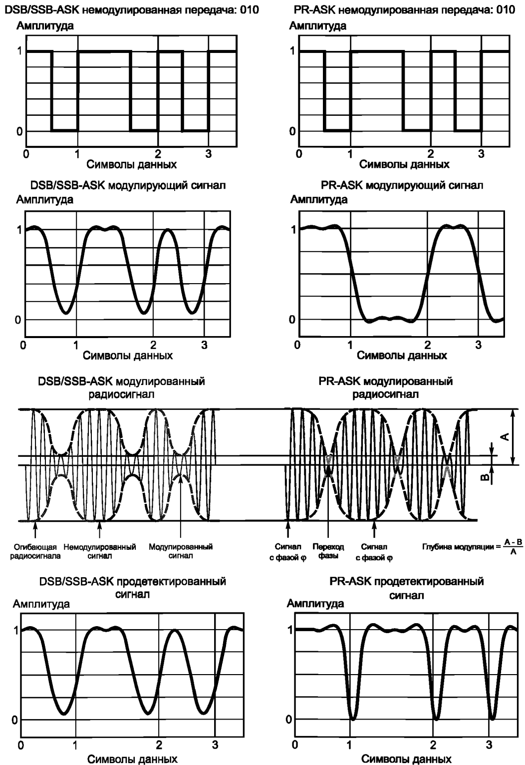
Рисунок Н.1 — Модуляция сигнала линии связи «устройство опроса — радиочастотная метка»
