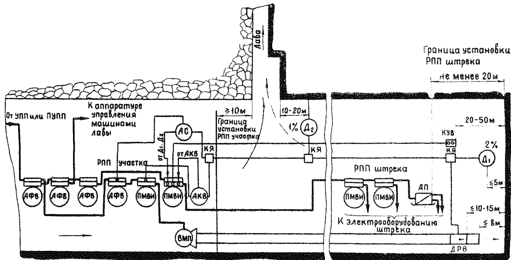
Рис. I. Схема электроснабжения и расстановки электрооборудования при проведении откаточного штрека
