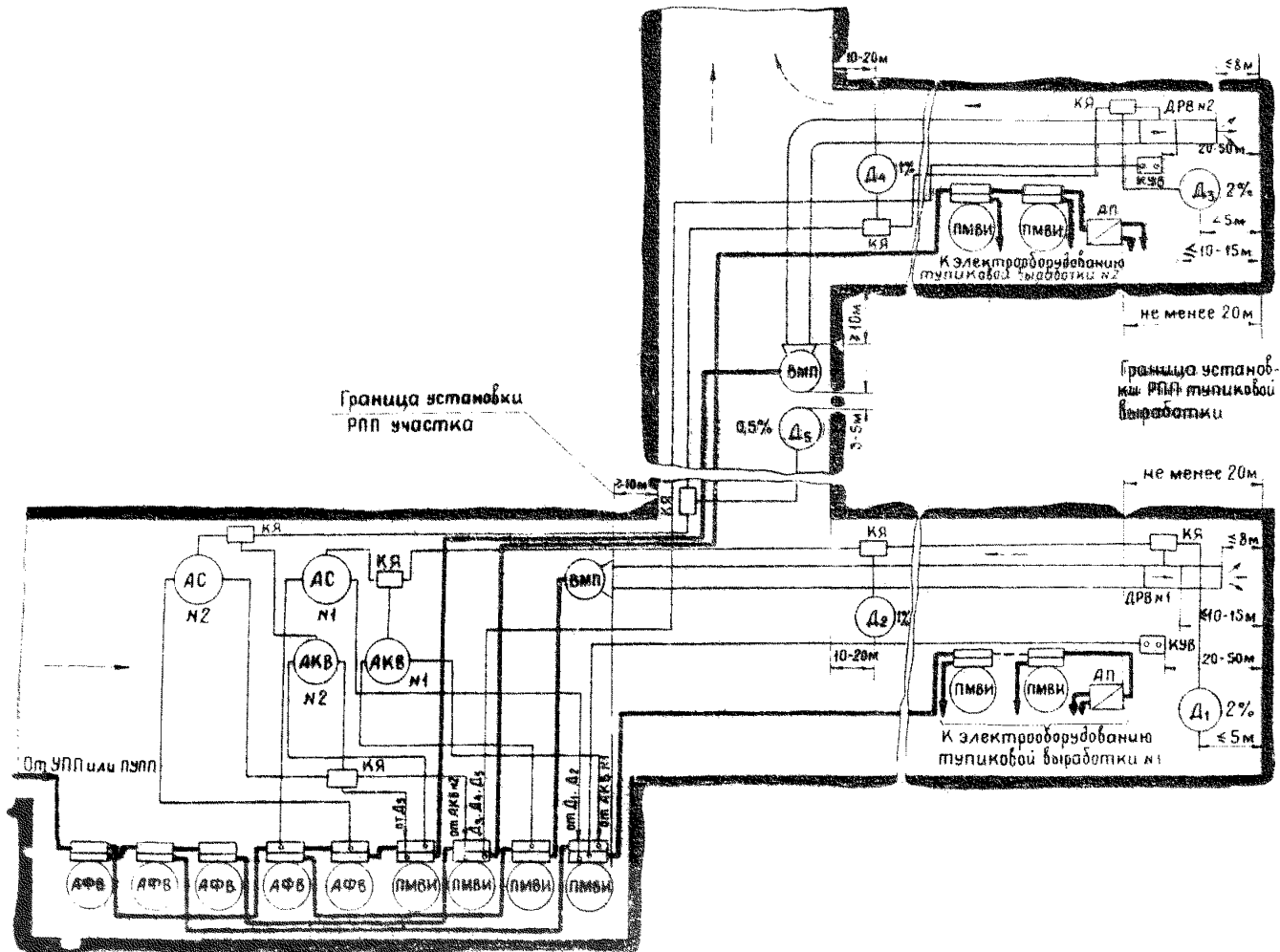
Рис. 4. Схема электроснабжения и восстановления электрооборудования в тупиковых выработках при установке ВПИ на исходящей струе
