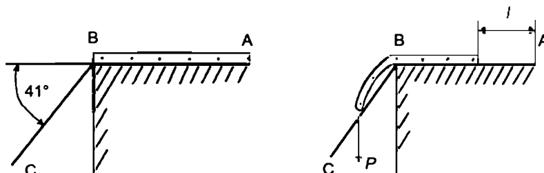
Рисунок А.1 – Схема измерения длины веревки
