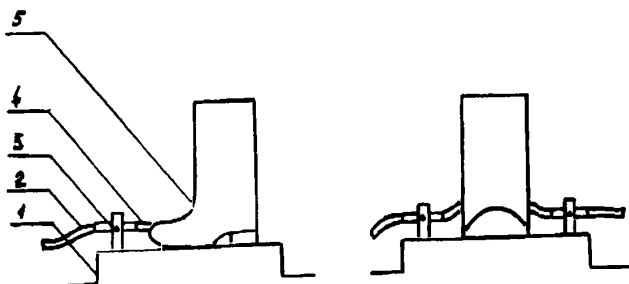
1 – станина; 2 – трубка подачи газа; 3 – горелка; 4 – открытое пламя; 5 – специальная защитная обувь
