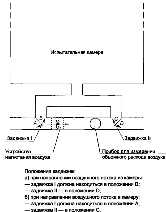
Рисунок A.2 — Схема испытательной камеры с системой подачи воздуха
