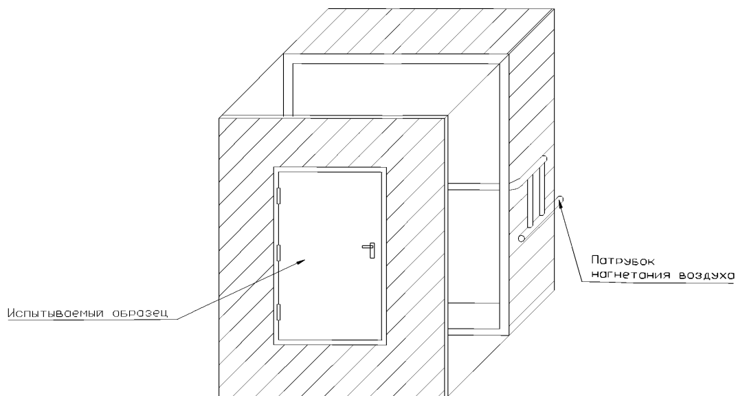
Рисунок А.1 — Схема испытательной камеры
