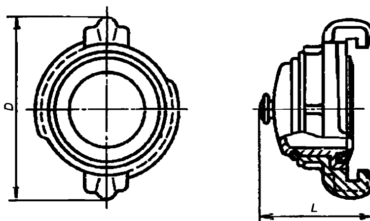
Рисунок 5 – Напорная головка типа ГЗ
